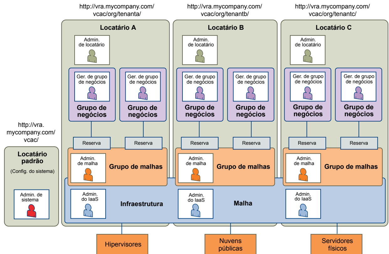
Figura 3. Exemplo de vários tenants com configuração de infraestrutura em cada tenant
