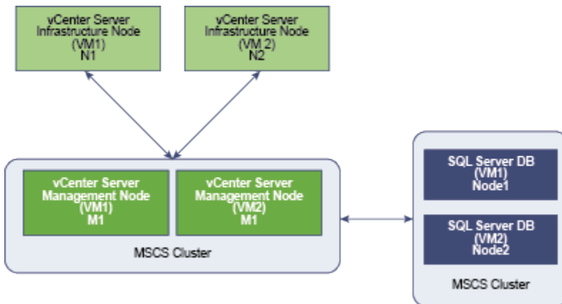
图 5-1 实现 vCenter Server 高可用性的 MSCS 群集
