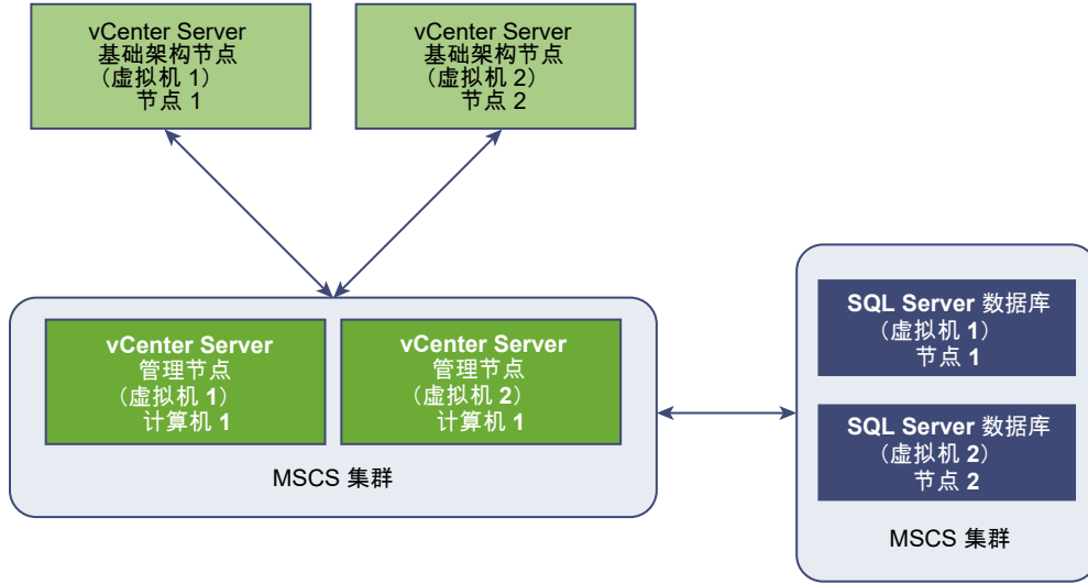
图 5-1. 实现 vCenter Server 高可用性的 MSCS 集群
