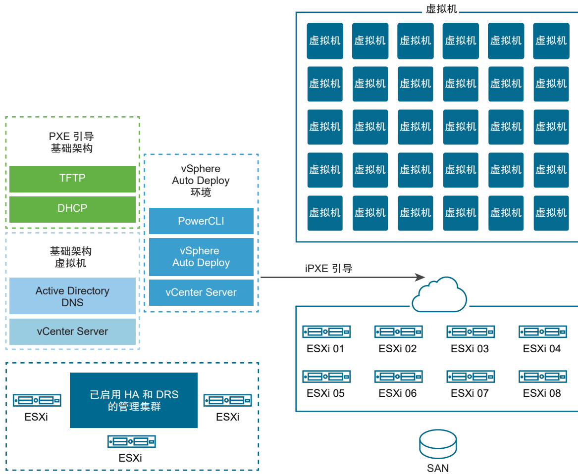
图 5-9. 具有高可用性的 vSphere Auto Deploy 基础架构
