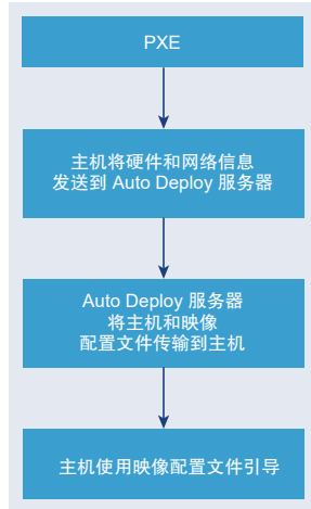
图 5-6. vSphere Auto Deploy 安装，首次引导
