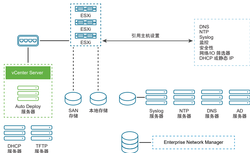
图 5-8. vSphere Auto Deploy 引用主机设置
