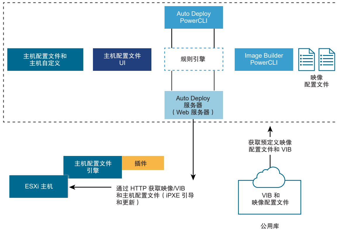
图 5-5. vSphere Auto Deploy 架构
