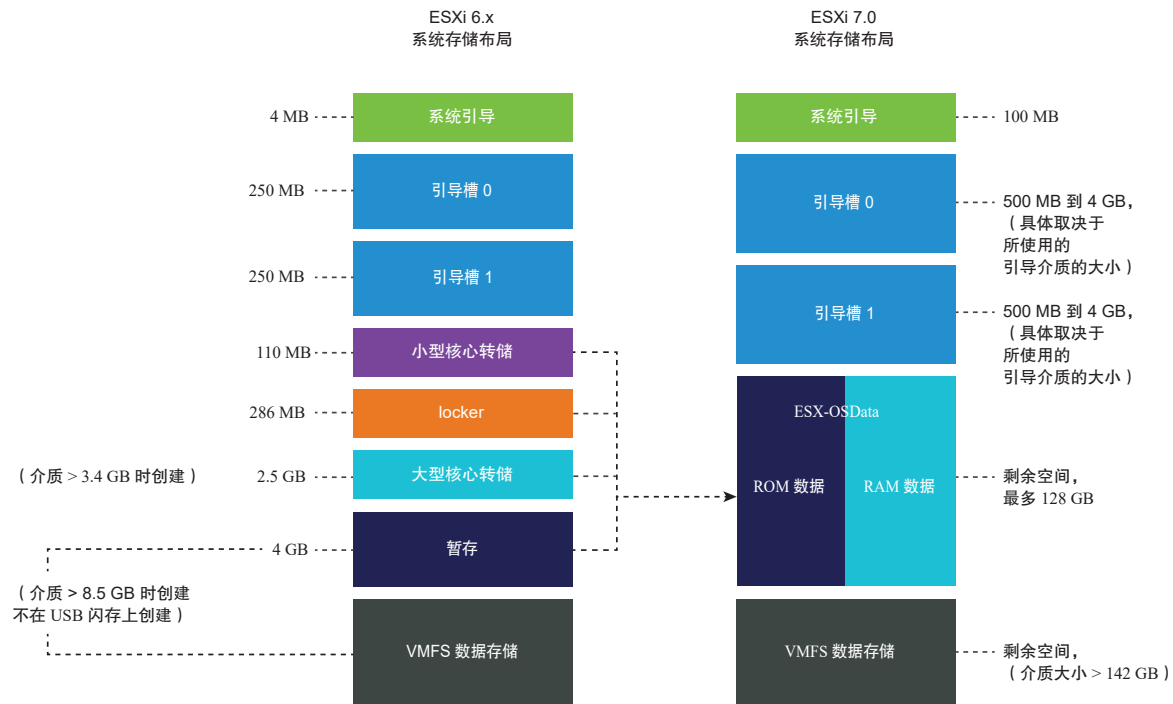
图 5-1. ESXi 7.0 及更高版本中整合的系统存储
