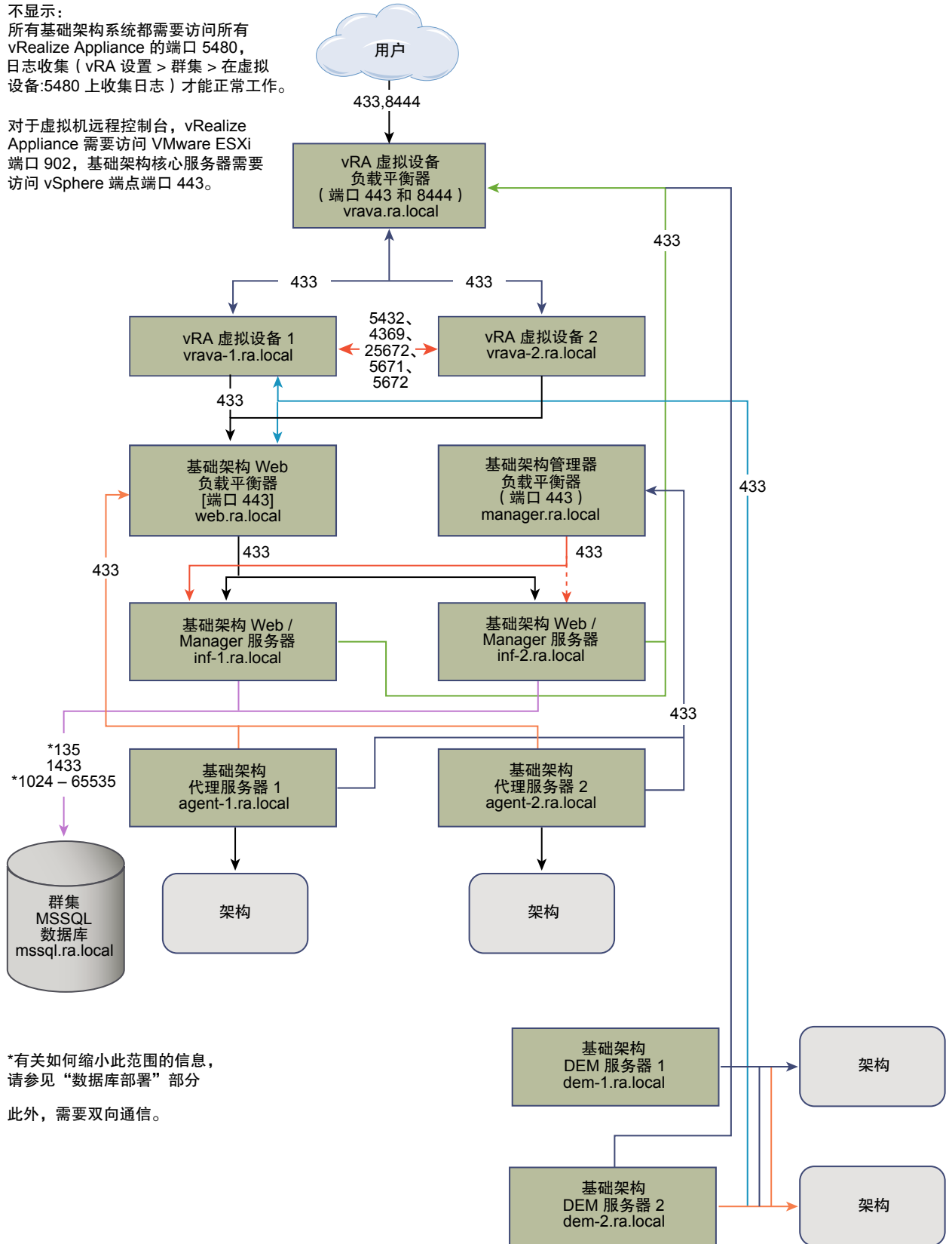
图 11-1 vRealize Automation 中型配置的最小占用空间
