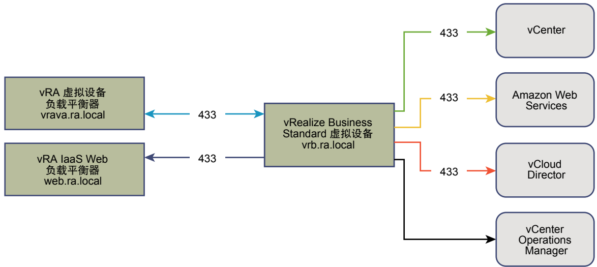
图 11-2 vRealize Business Standard Edition 中型部署的最小占用空间
