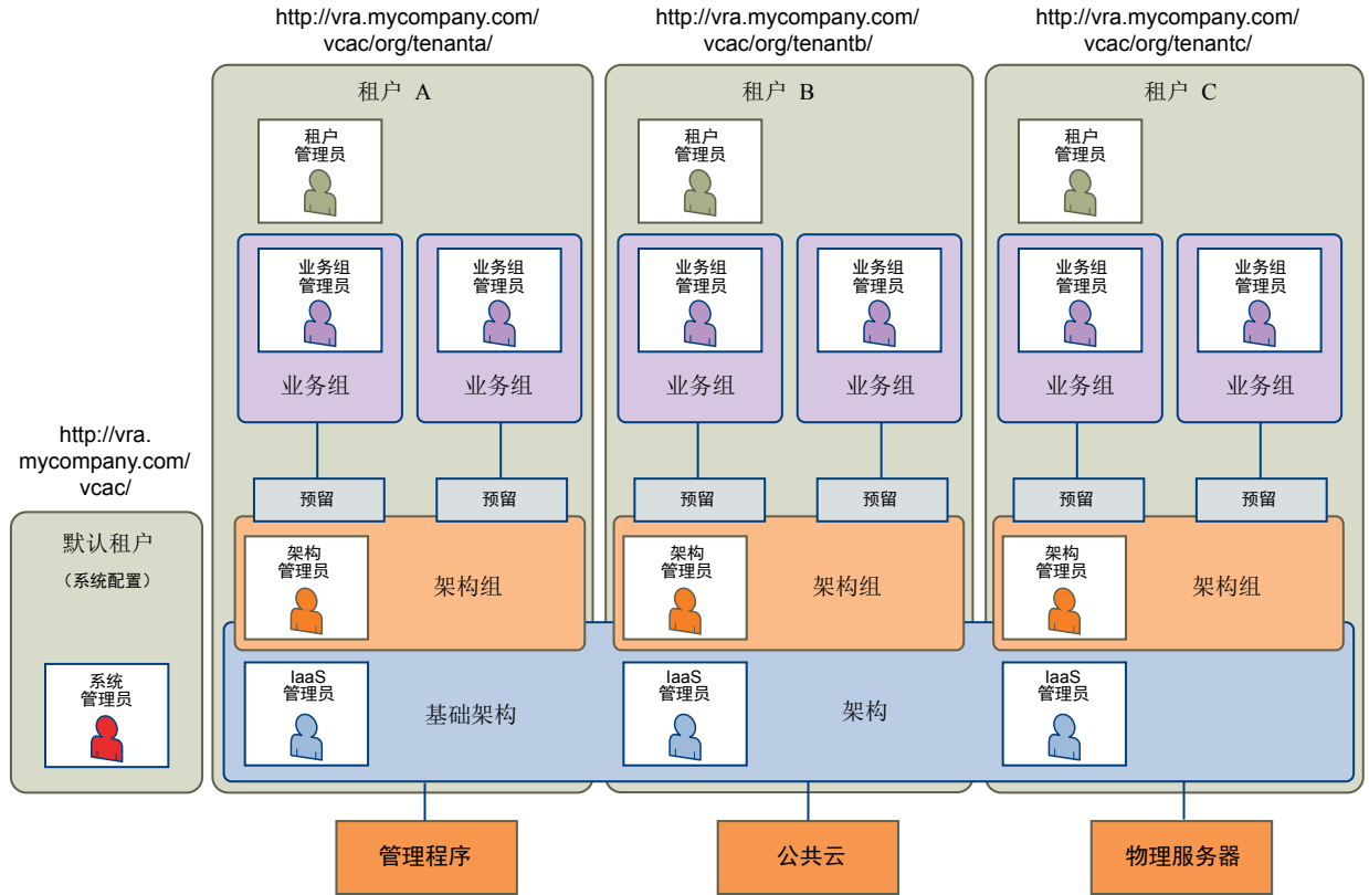
图 3 每个租户中包含基础架构配置的多租户示例
