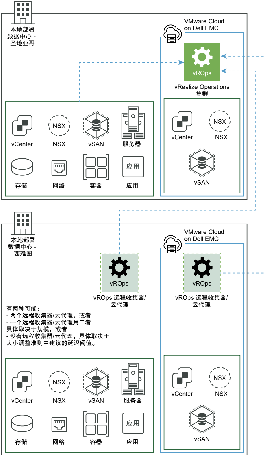
图 3-15. VMware Cloud 中的 VMware Cloud on Dell EMC 使用或不使用远程数据收集器从 vRealize Operations 和内部部署收集数据
