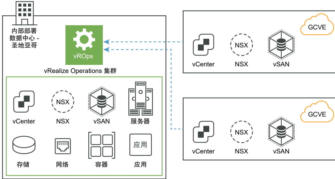
图 3-13. vRealize Operations 本地部署在不使用远程数据收集器的情况下从 Google Cloud VMware Engine 收集数据
