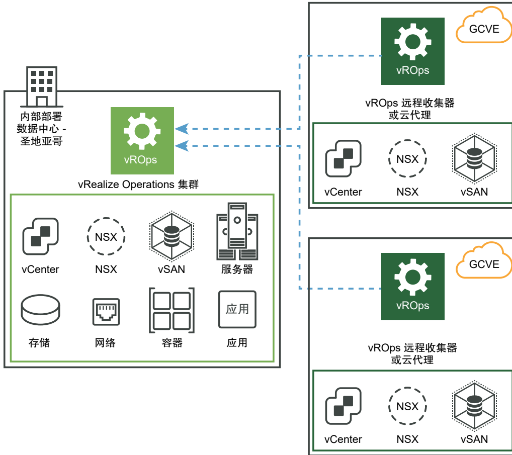
图 3-12. (建议) vRealize Operations 内部部署使用远程数据收集器从 Google Cloud VMware Engine 收集数据
