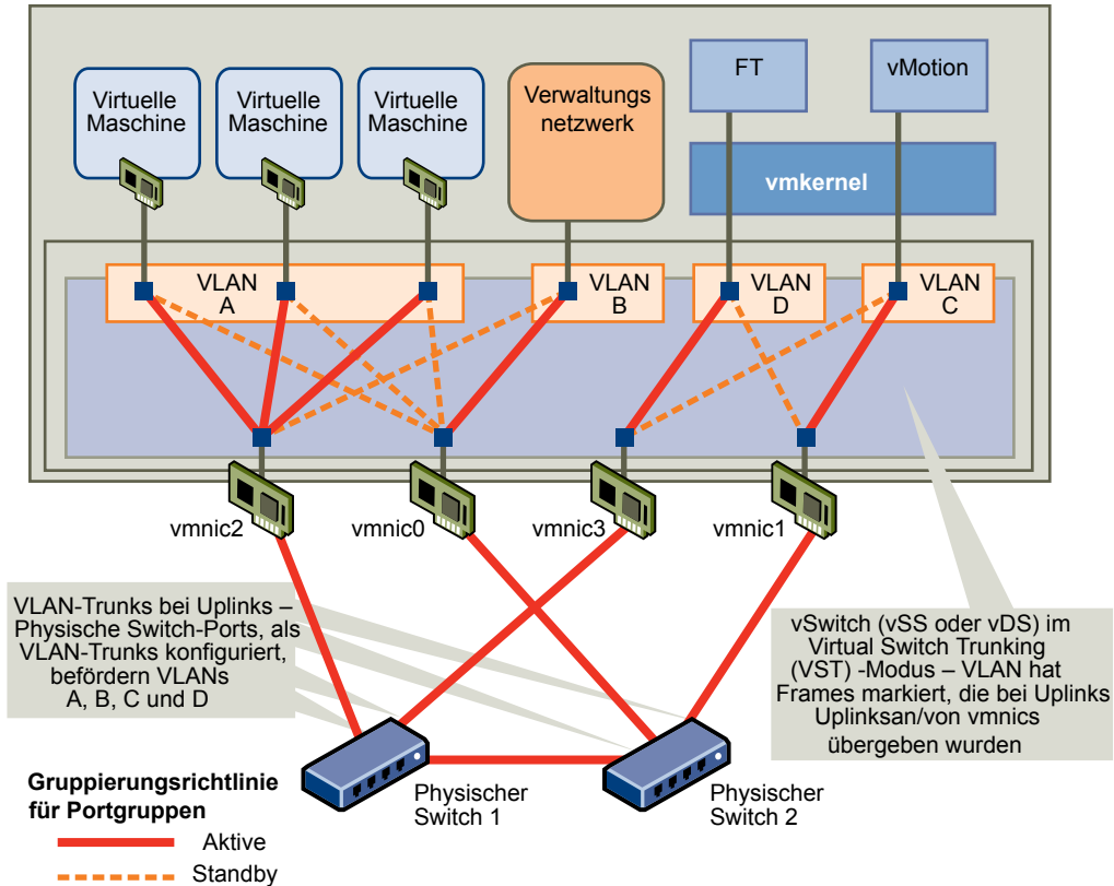
Abbildung 3-2. Fault Tolerance - Beispiel einer Netzwerkkonfiguration
