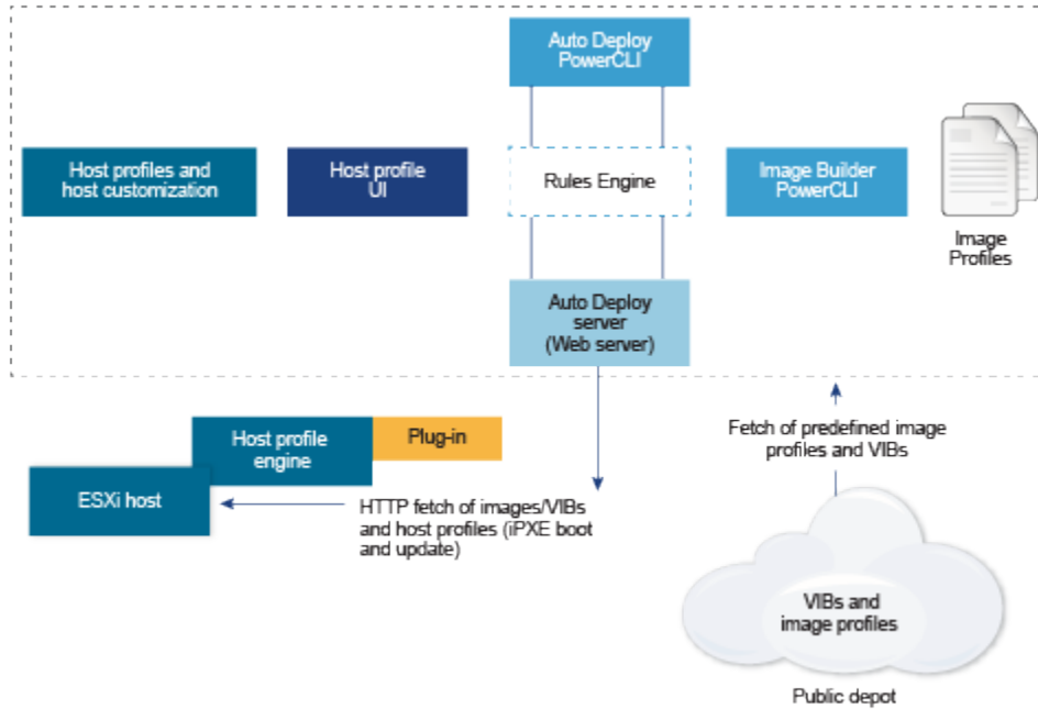
Abbildung 2-4. vSphere Auto Deploy-Architektur
