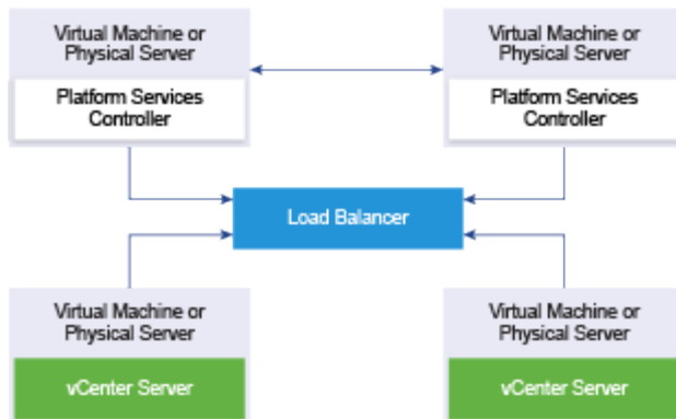
Abbildung 1-6. Beispiel für ein Paar von Platform Services Controller -Instanzen mit Lastausgleich
