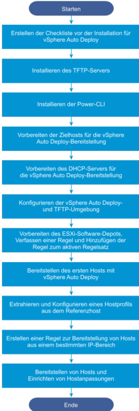
Abbildung 2-9. Workflow für das Setup von vSphere Auto Deploy und die Hostbereitstellung
