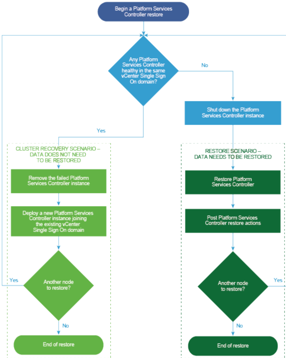
Abbildung 7-2. Platform Services Controller -Wiederherstellungs-Workflow
