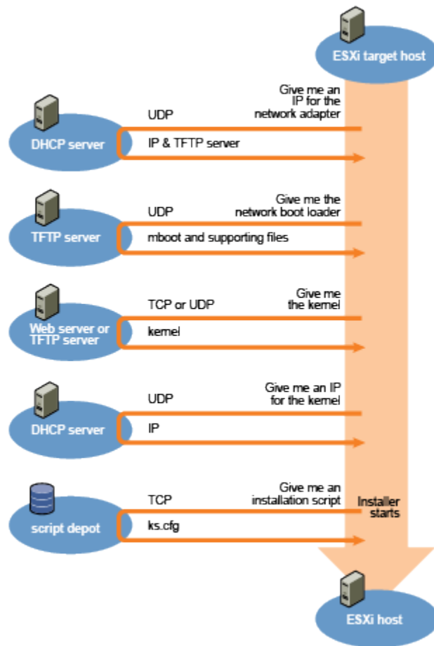
Abbildung 2-3. Überblick über den Installationsprozess per PXE-Startvorgang
