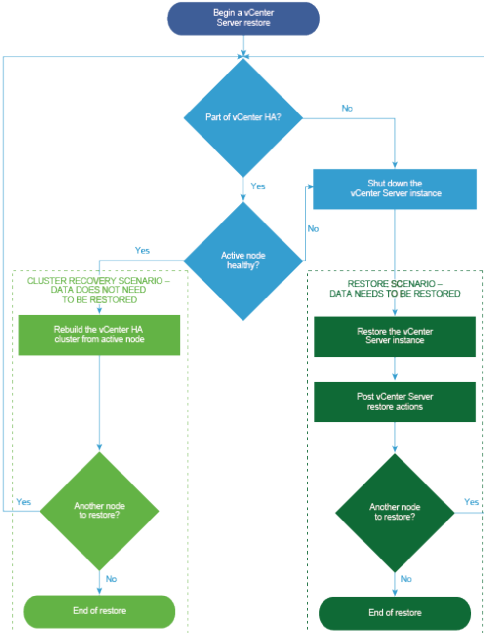
Abbildung 7-1. vCenter Server -Wiederherstellungs-Workflow
