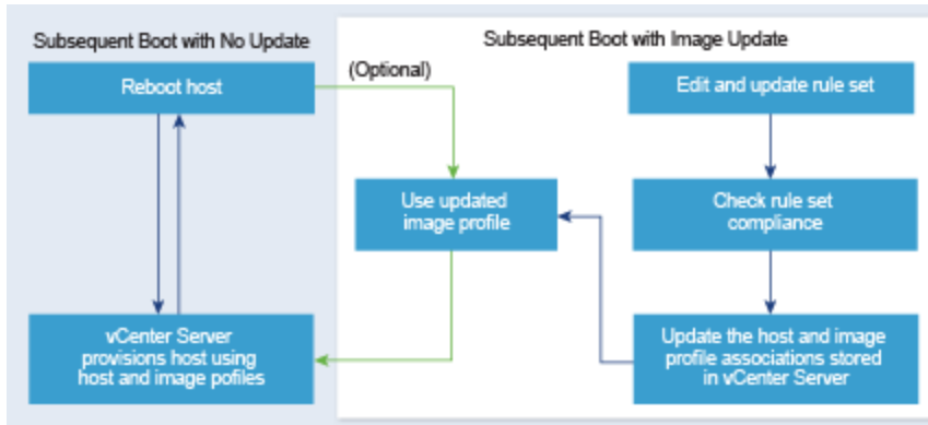
Abbildung 2-6. vSphere Auto Deploy-Installation, nachfolgende Starts
