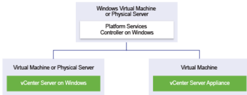
Abbildung 1-4. Beispiel einer Umgebung mit gemischten Betriebssystemen mit einem externen Platform Services Controller unter Windows
