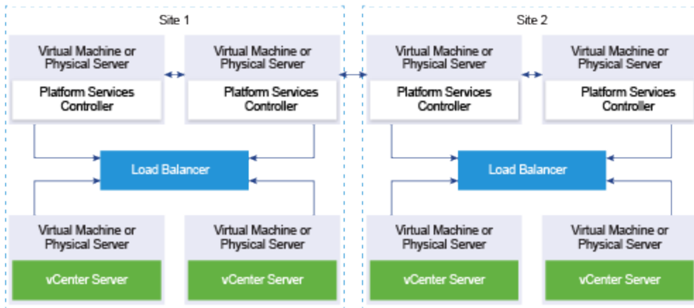
Abbildung 1-7. Beispiel für zwei Platform Services Controller -Instanzen mit Lastausgleich zwischen zwei Sites
