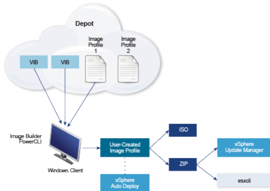
Abbildung 2-2. Image Builder-Architektur
