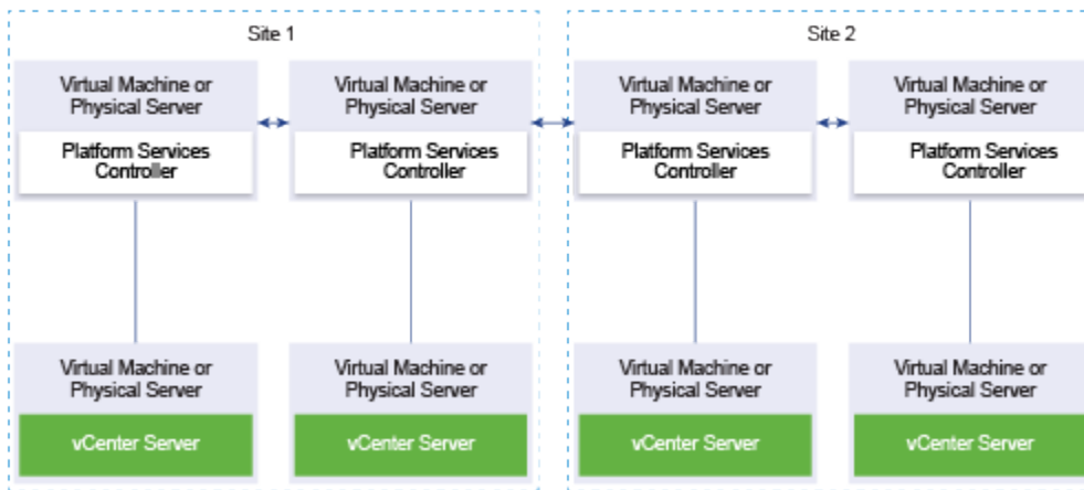
Abbildung 1-9. Beispiel für zwei hinzugefügte Paare von Platform Services Controller -Instanzen zwischen zwei Sites ohne Lastausgleichsdienst
