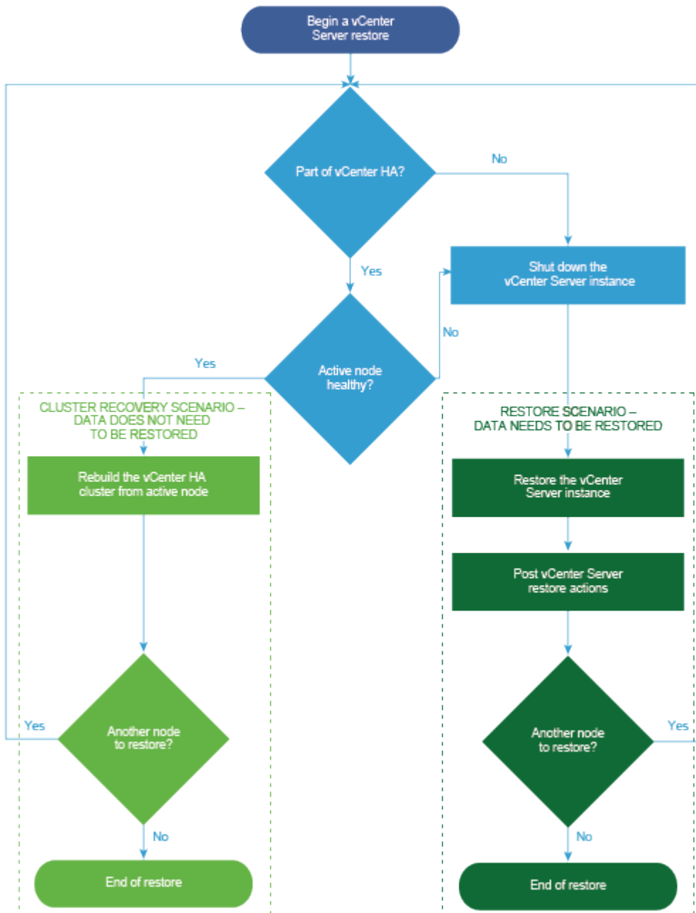
Abbildung 6-1. vCenter Server Appliance -Wiederherstellungs-Workflow
