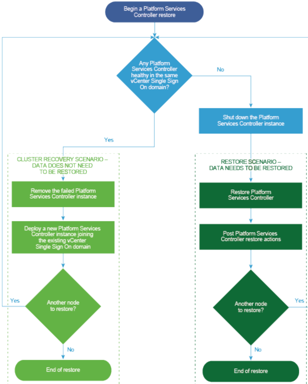
Abbildung 6-2. Wiederherstellungs-Workflow der Platform Services Controller -Appliance
