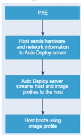
Abbildung 2-5. vSphere Auto Deploy-Installation, erster Start
