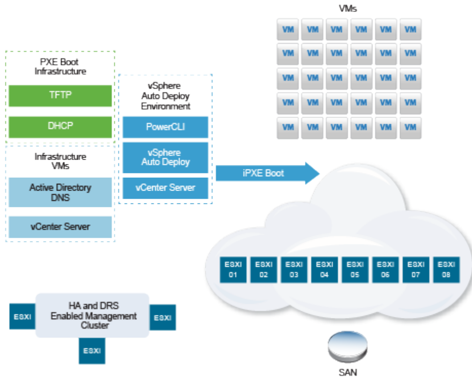
Abbildung 2-8. vSphere Auto Deploy-Infrastruktur für hohe Verfügbarkeit
