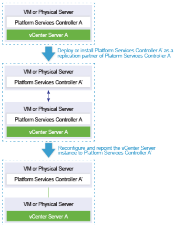
Abbildung 5-1. Neukonfigurieren einer eigenständigen vCenter Server-Instanz mit einem eingebetteten Platform Services Controller und Neuverweisen der Instanz auf einen externen Platform Services Controller
