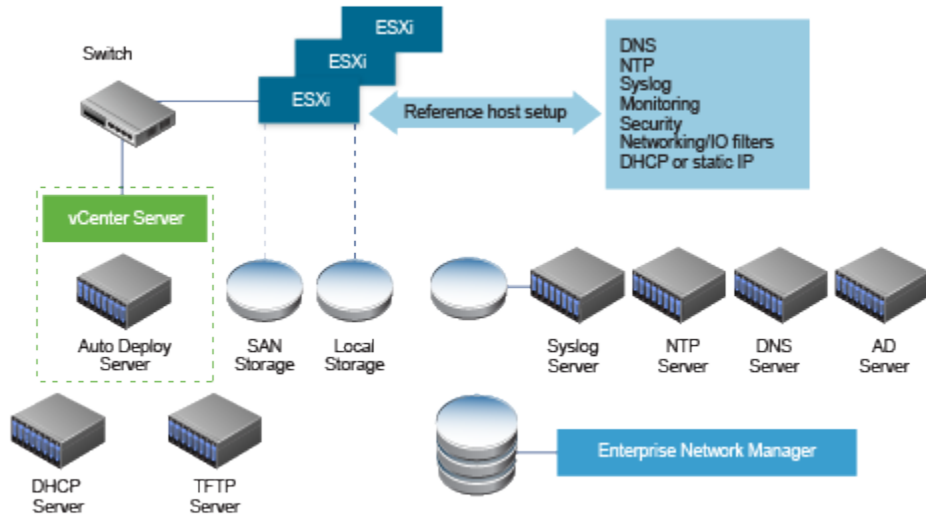
Abbildung 2-7. vSphere Auto Deploy-Referenzhost-Einrichtung
