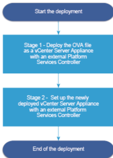
Abbildung 3-5. Bereitstellungs-Workflow von vCenter Server Appliance mit einem externen Platform Services Controller
