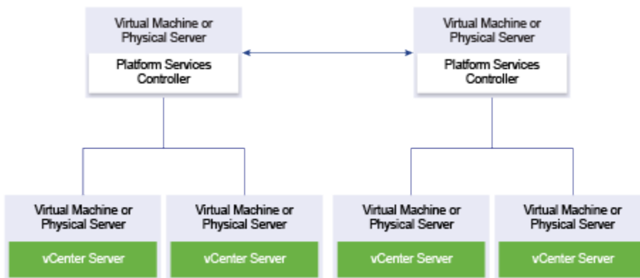
Abbildung 1-8. Beispiel für zwei hinzugefügte Platform Services Controller -Instanzen ohne Lastausgleichsdienst
