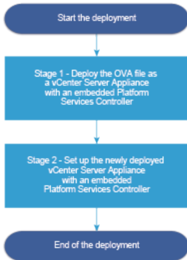
Abbildung 3-3. Bereitstellungs-Workflow einer vCenter Server Appliance mit einem eingebetteten Platform Services Controller
