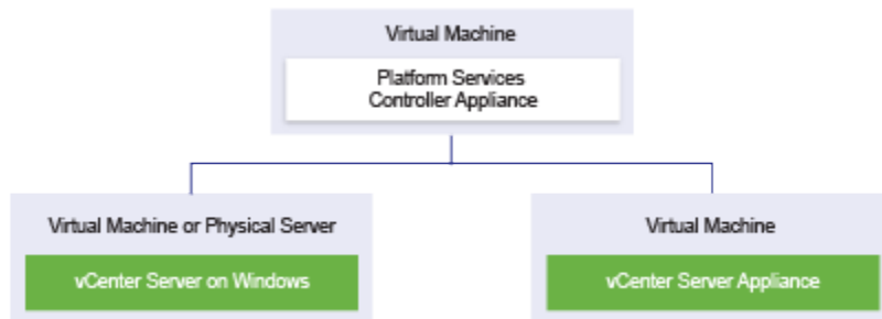
Abbildung 1-5. Beispiel einer Umgebung mit gemischten Betriebssystemen mit einer externen Platform Services Controller-Appliance
