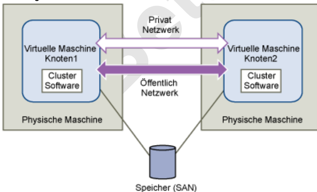
Abbildung 1-2. Virtuelle Maschinen in Clustern auf mehreren Hosts
