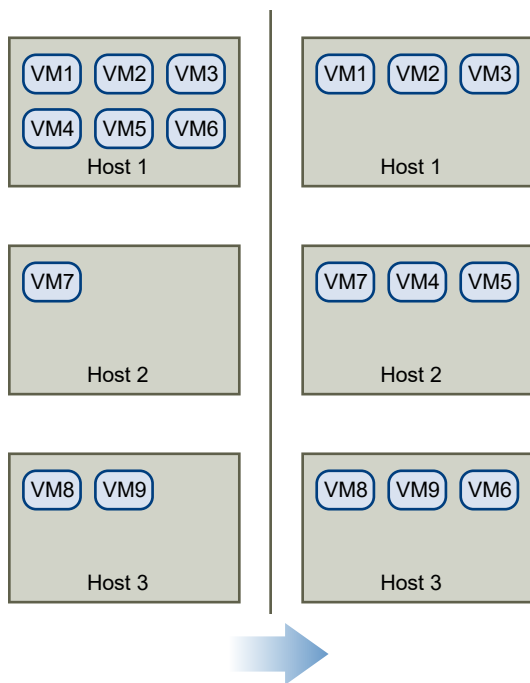
Abbildung 11-1. Lastenausgleich
