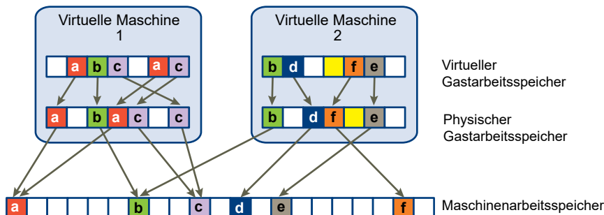
Abbildung 9-2. Beispiel für die Arbeitsspeichernutzung
