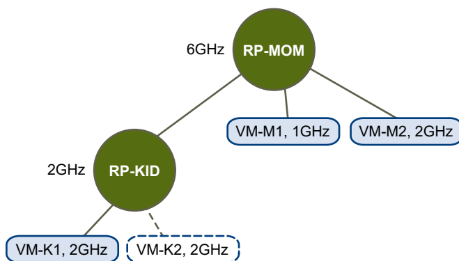
Abbildung 14-4. Zugangssteuerung bei erweiterbaren Ressourcenpools: Einschalten verhindert
