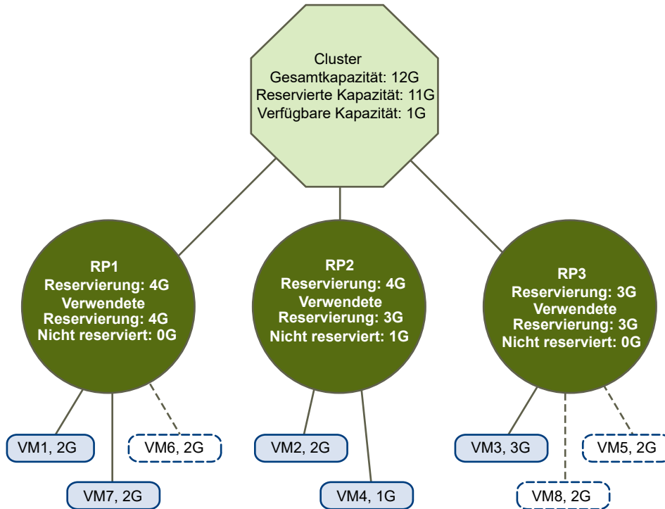
Abbildung 18-1. Gültiger Cluster mit festen Ressourcenpools
