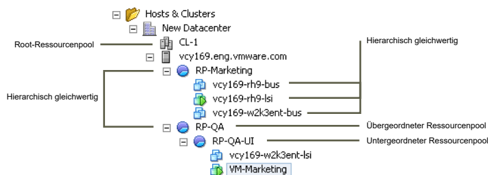
Abbildung 14-1. Übergeordnete, untergeordnete und hierarchisch gleichwertige Ressourcenpools in der Ressourcenpoolhierarchie
