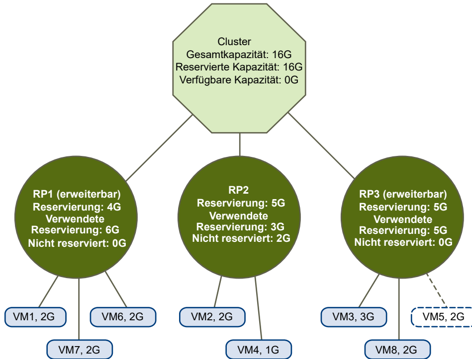
Abbildung 18-2. Gültiger Cluster mit erweiterbaren Ressourcenpools
