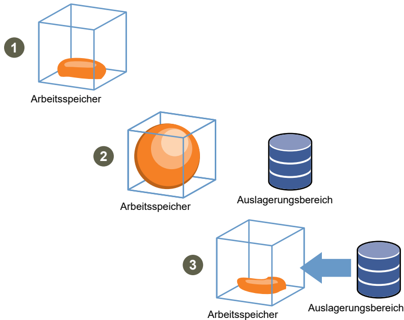
Abbildung 9-1. Arbeitsspeicher-Ballooning im Gastbetriebssystem
