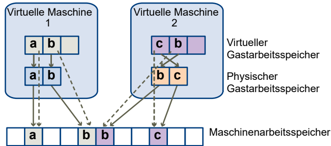
Abbildung 8-1. Arbeitsspeicherzuordnung bei ESXi
