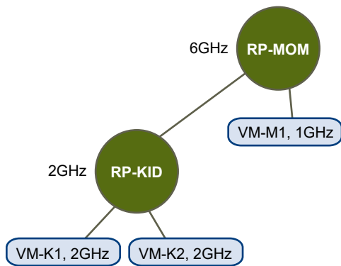
Abbildung 14-3. Zugangssteuerung bei erweiterbaren Ressourcenpools: Einschalten erfolgreich
