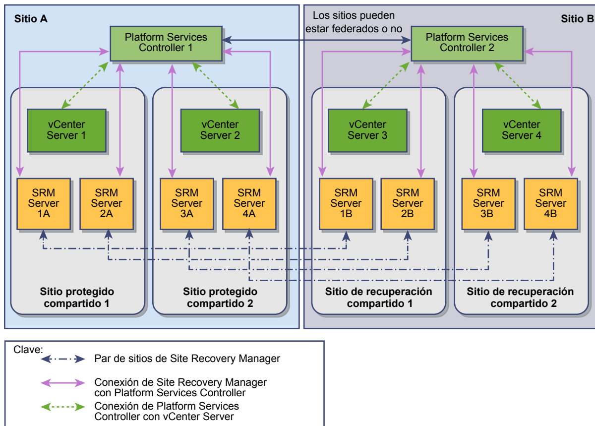
Figura 10-3. Site Recovery Manager en un sitio protegido compartido y una configuración de sitio de recuperación compartido
