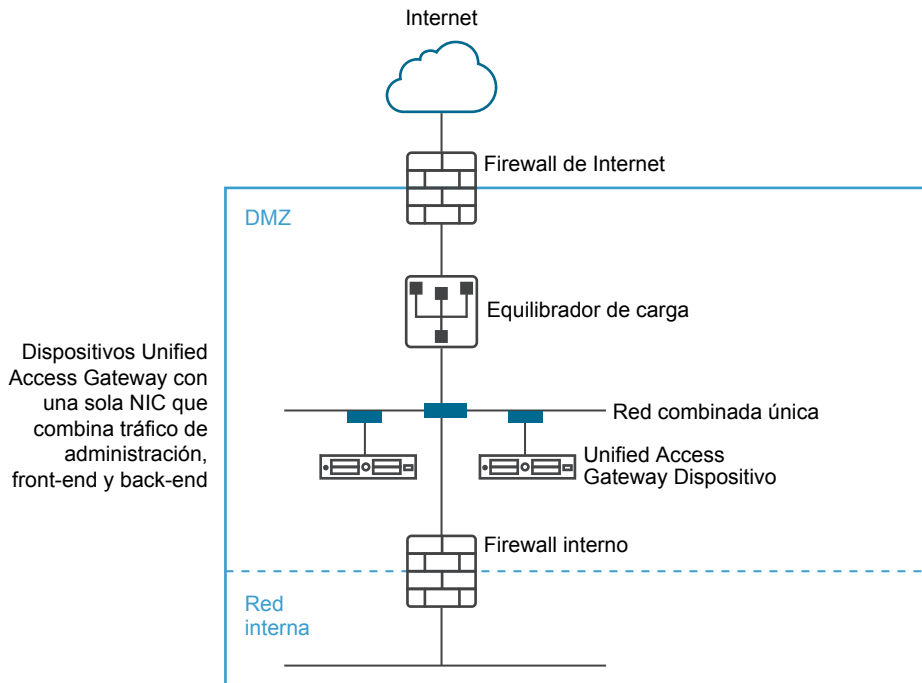
Figura 1-3. Unified Access Gateway con una sola NIC
