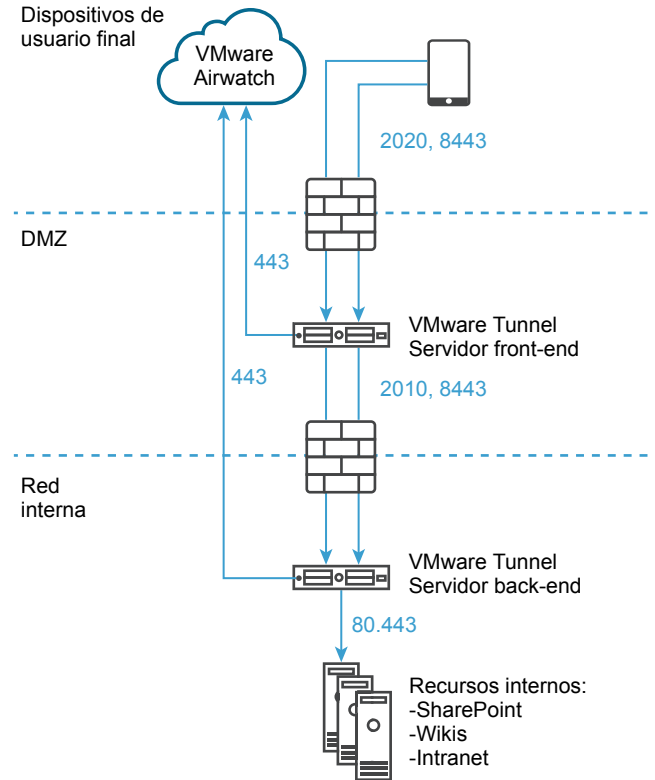
Figura 4-8. Implementación de varios niveles de VMware Tunnel: proxy y túnel por aplicación
