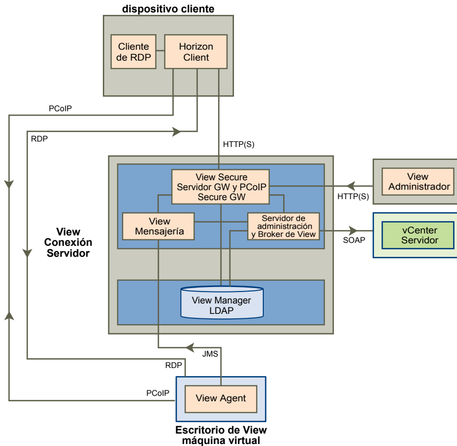
Figura 5-5. Componentes y protocolos de View sin un servidor de seguridad
