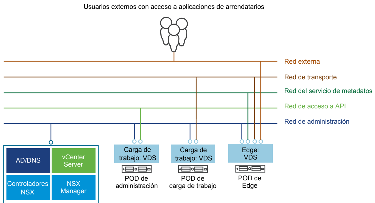
Figura 2-4. Mapa de red para las implementaciones de NSX
