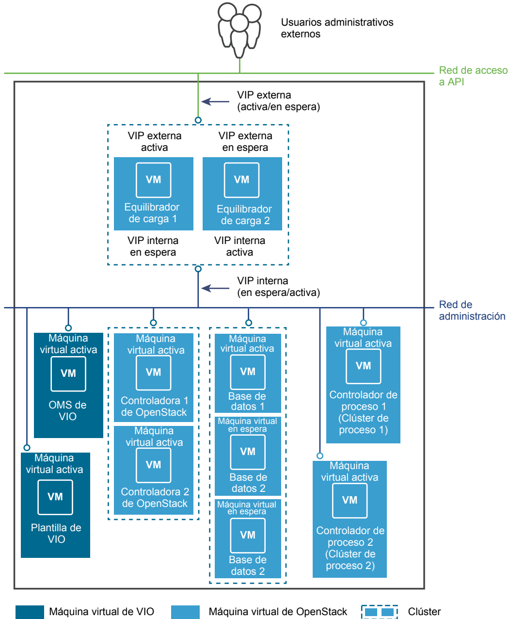
Figura 2-2. Clúster de administración en modo HA
