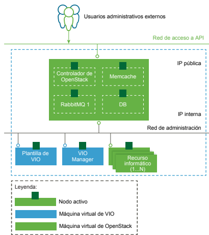
Figura 4-1. Clúster de administración en modo compacto
