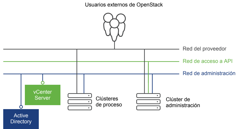
Figura 3-1. VMware Integrated OpenStack : Red física de VDS
