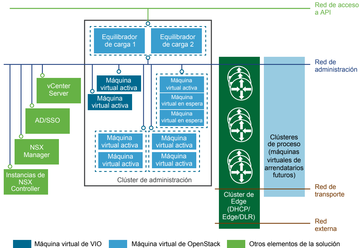
Figura 2-1. Implementación de NSX en modo HA
