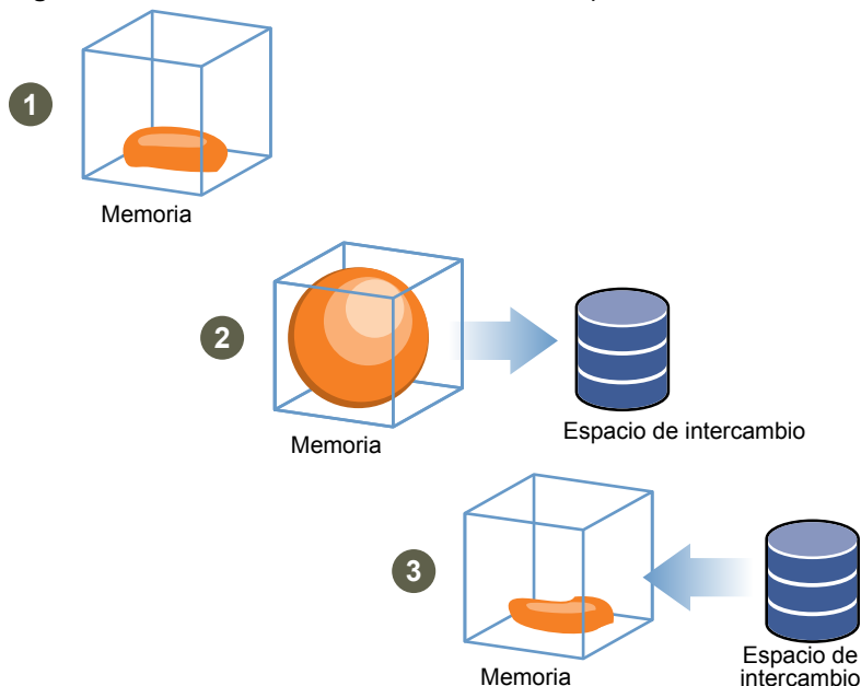
Figura 6-1. Aumentar la memoria en el sistema operativo invitado
