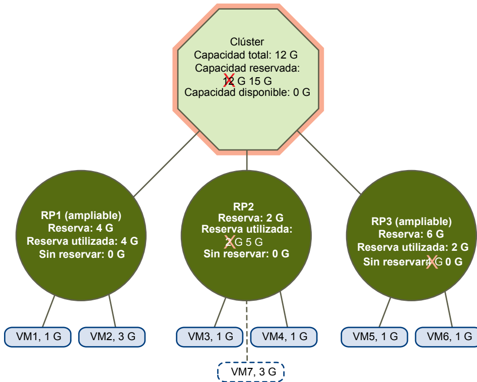
Figura 11-4. clúster rojo
