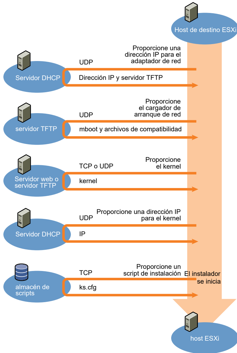
Figura 3-1. Descripción general de la instalación del arranque PXE
