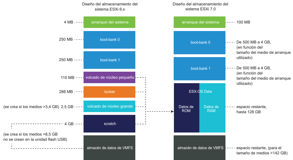
Figura 5-1. Almacenamiento consolidado del sistema en ESXi 7.0 y versiones posteriores
