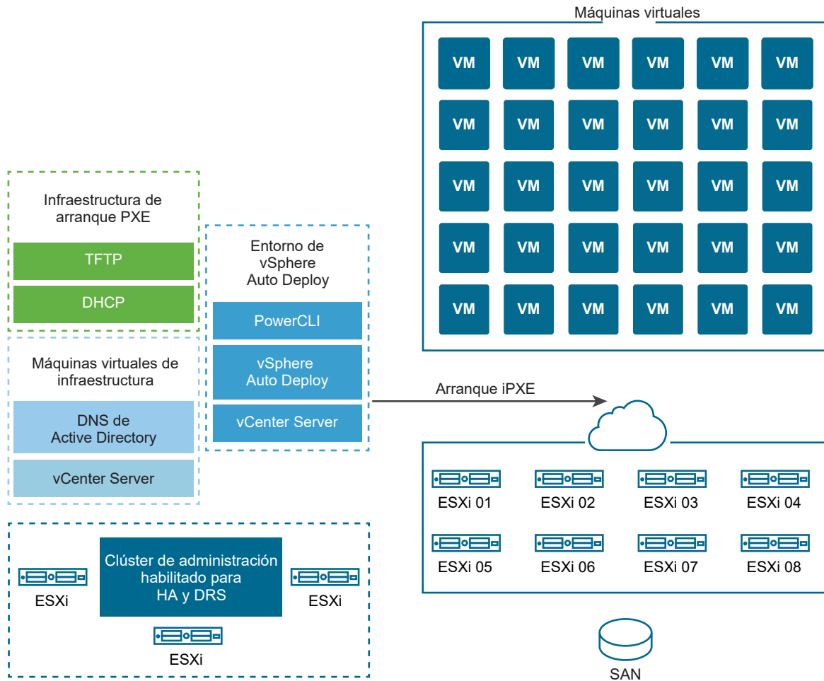
Figura 5-9. Infraestructura de vSphere Auto Deploy de alta disponibilidad
