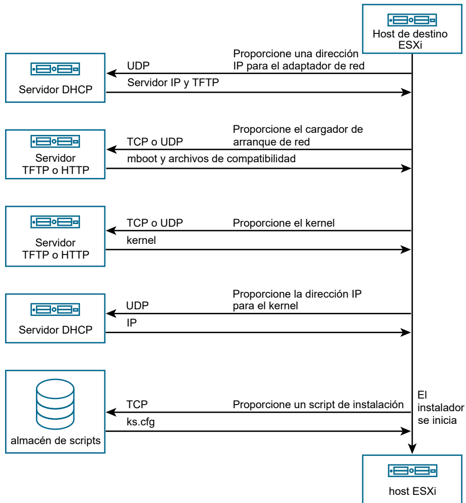
Figura 5-4. Descripción general de la instalación del arranque PXE
