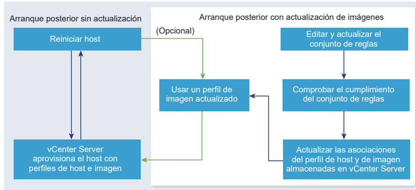
Figura 5-7. Instalación de vSphere Auto Deploy, arranques posteriores
