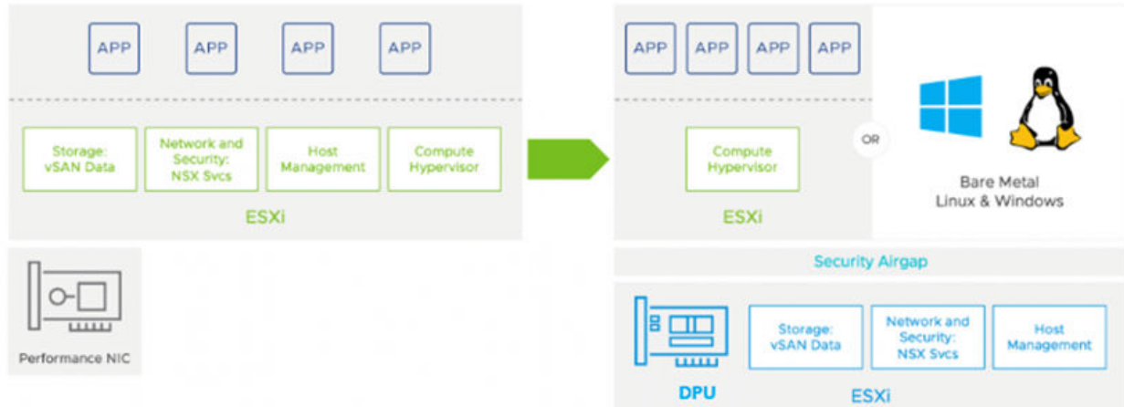
Figura 3-1. A partir de vSphere 8.0, VMware traslada cierta funcionalidad que se ejecuta en el complejo de CPU principal al complejo de CPU de DPU:
