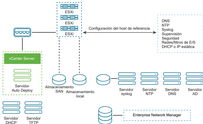
Figura 4-8. Configurar el host de referencia con vSphere Auto Deploy
