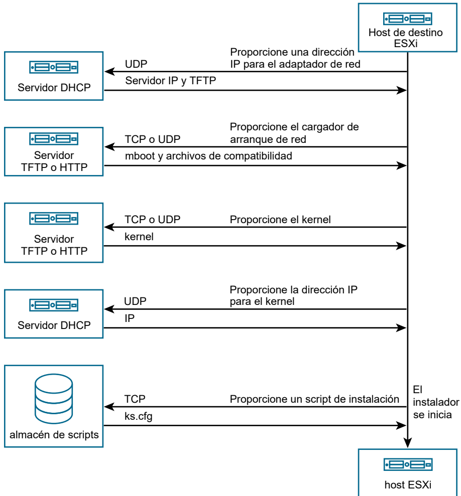
Figura 4-4. Descripción general de la instalación del arranque PXE
