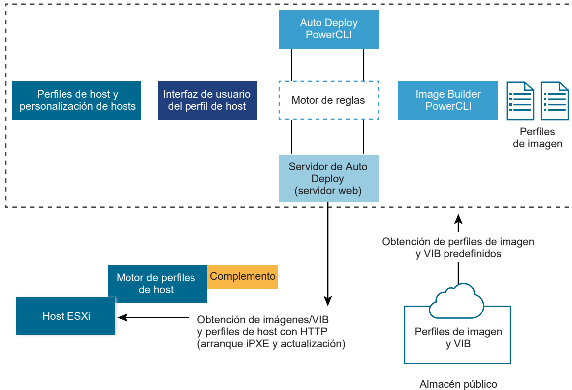
Figura 4-5. Arquitectura de vSphere Auto Deploy
