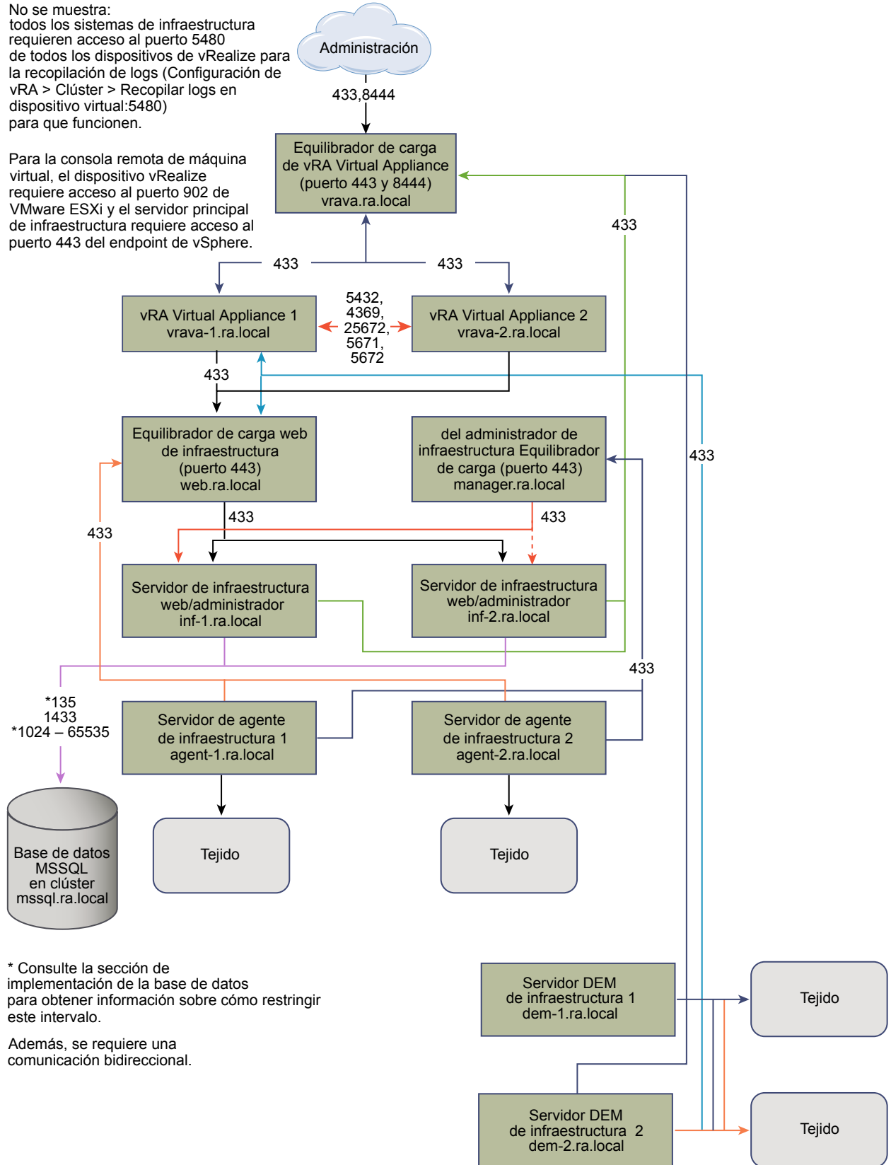
Figura 11-1. Huella mínima para configuración mediana de vRealize Automation
