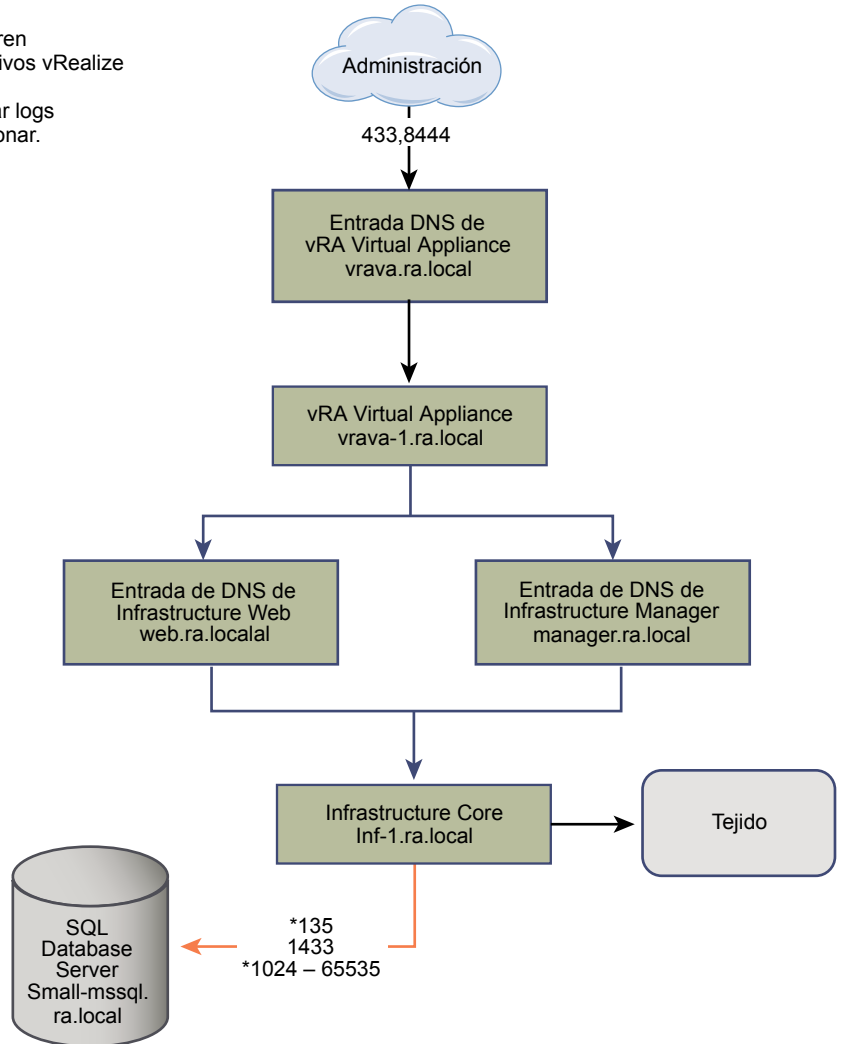
Figura 10-1. Huella mínima para una configuración pequeña de vRealize Automation
