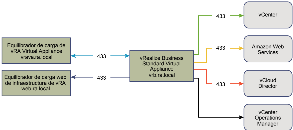
Figura 12-2. Huella mínima para configuración mayor de vRealize Business Standard Edition
