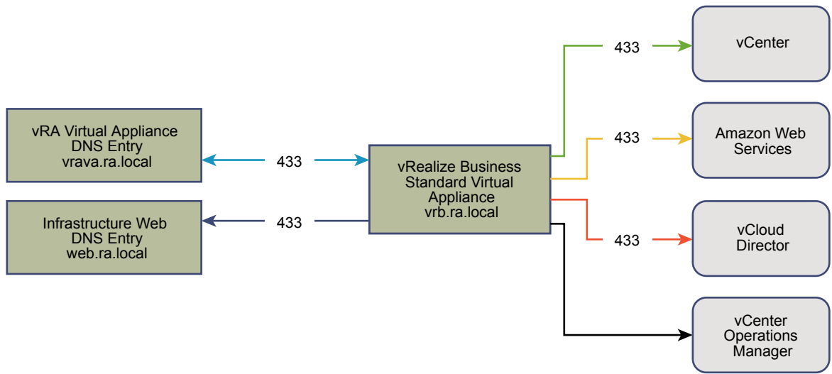
Figura 10-2. Huella mínima para una configuración pequeña de vRealize Business Standard Edition
