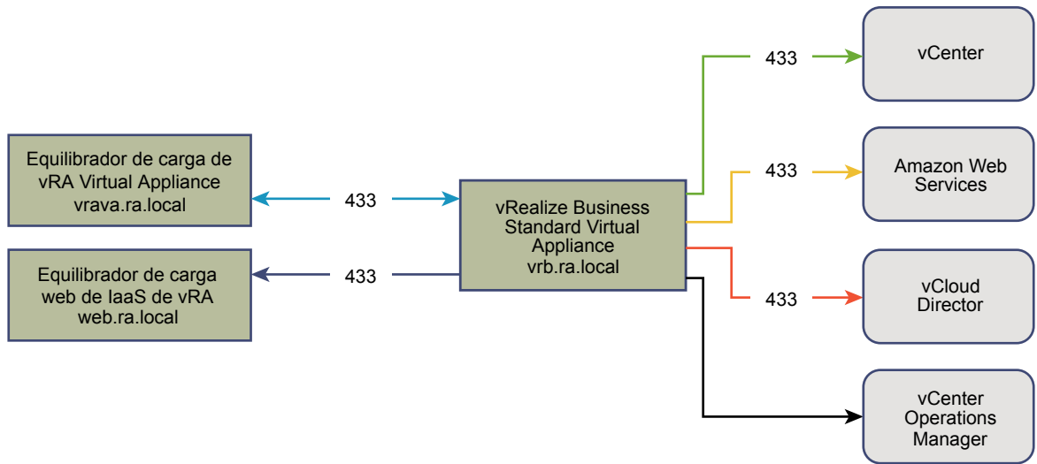
Figura 11-2. Huella mínima para configuración mediana de vRealize Business Standard Edition
