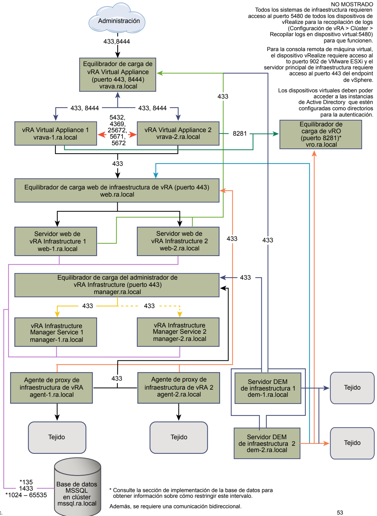
Figura 12-1. Huella mínima para configuración mayor de vRealize Automation
