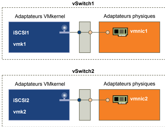
Figure 4-2. mappage d'adaptateurs 1:1 sur les commutateurs standards vSphere distincts
