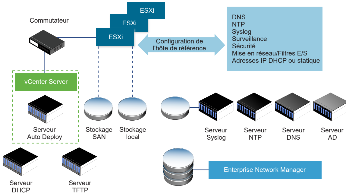
Figure 2-7. Configuration de l'hôte de référence vSphere Auto Deploy
