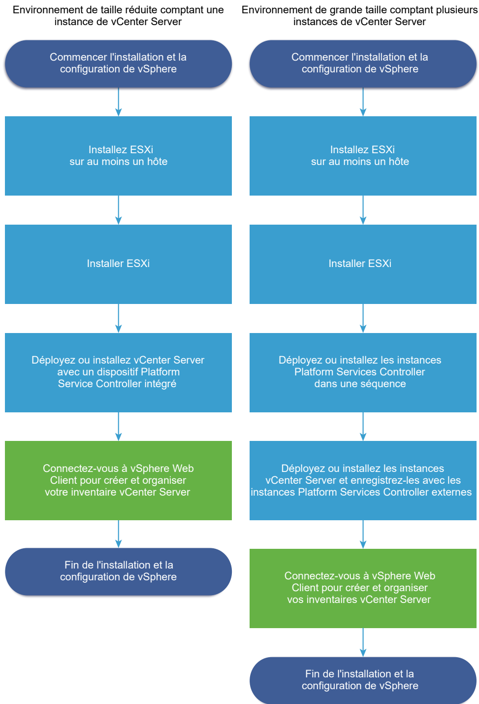
Figure 1-1. Workflow d'installation et de configuration de vSphere
