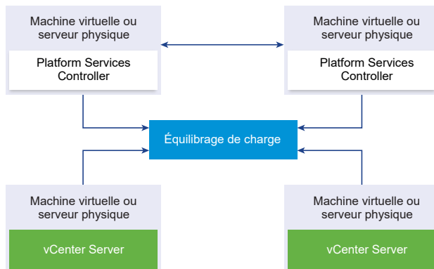
Figure 1-6. Exemple d'une paire d'instances de Platform Services Controller à charge équilibrée
