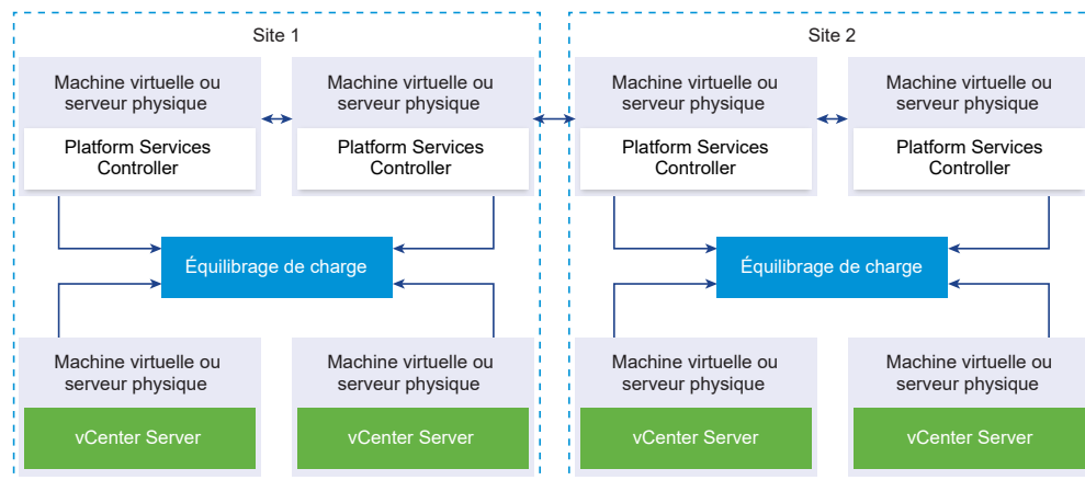
Figure 1-7. Exemple de deux paires d'instances de Platform Services Controller à charge équilibrée entre deux sites
