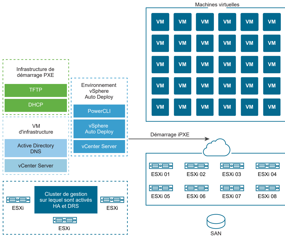
Figure 5-8. Infrastructure vSphere Auto Deploy à haute disponibilité
