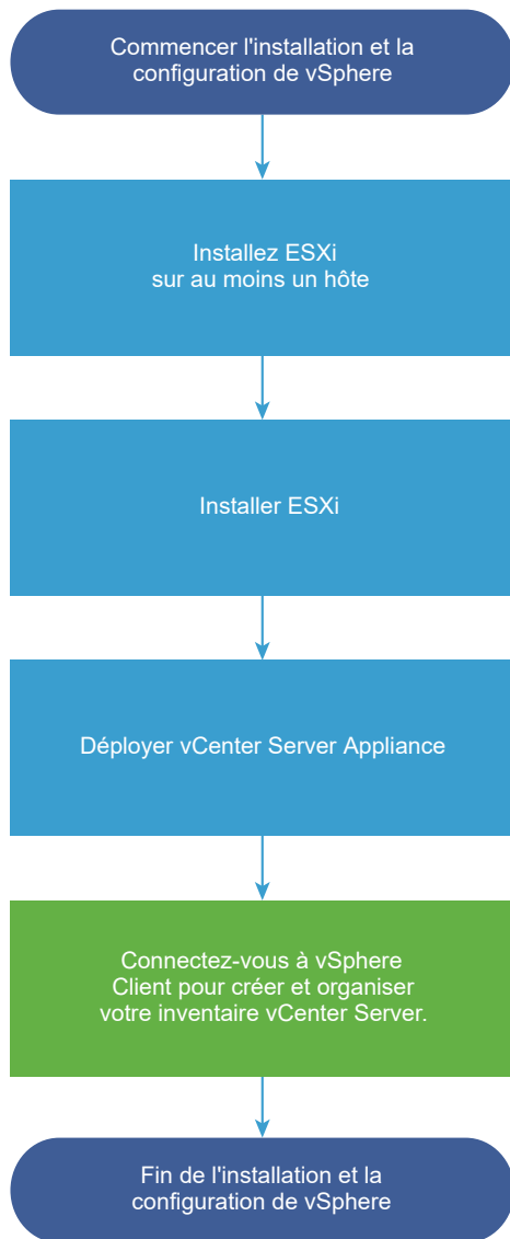
Figure 3-1. Workflow d'installation et de configuration de vSphere
