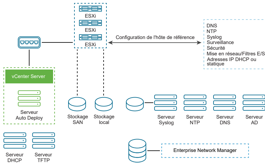
Figure 5-7. Configuration de l'hôte de référence vSphere Auto Deploy
