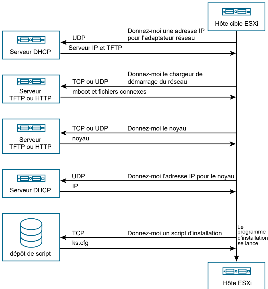
Figure 5-3. Présentation du processus d'installation du démarrage PXE
