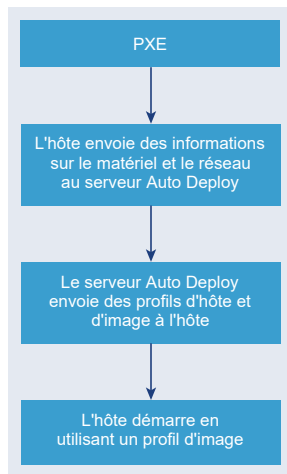
Figure 5-5. Installation de vSphere Auto Deploy, premier démarrage
