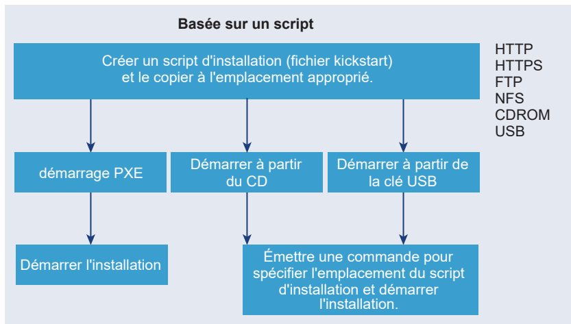
Figure 5-1. Installation en utilisant un script
