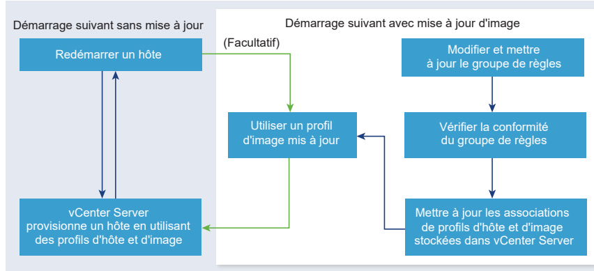
Figure 5-6. Installation de vSphere Auto Deploy, démarrages suivants
