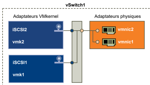
Figure 11-2. Mappage d'adaptateurs 1:1 sur un seul commutateur standard vSphere
