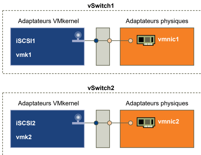
Figure 11-1. Mappage d'adaptateurs 1:1 sur des commutateurs standard vSphere distincts
