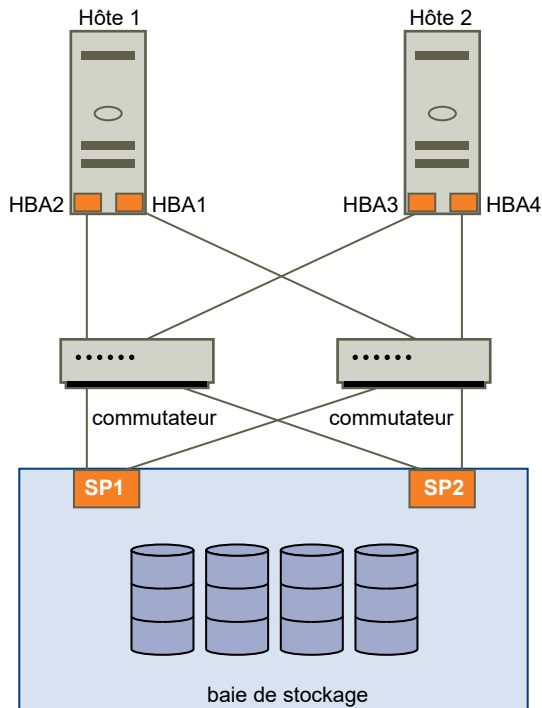
Figure 18-1. Gestion multivoie et basculement avec Fibre Channel
