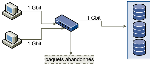
Figure 13-2. Paquets abandonnés
