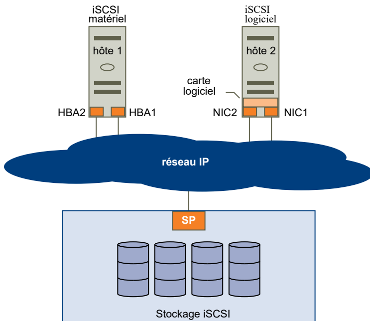
Figure 18-2. Basculement de chemin basé sur hôte
