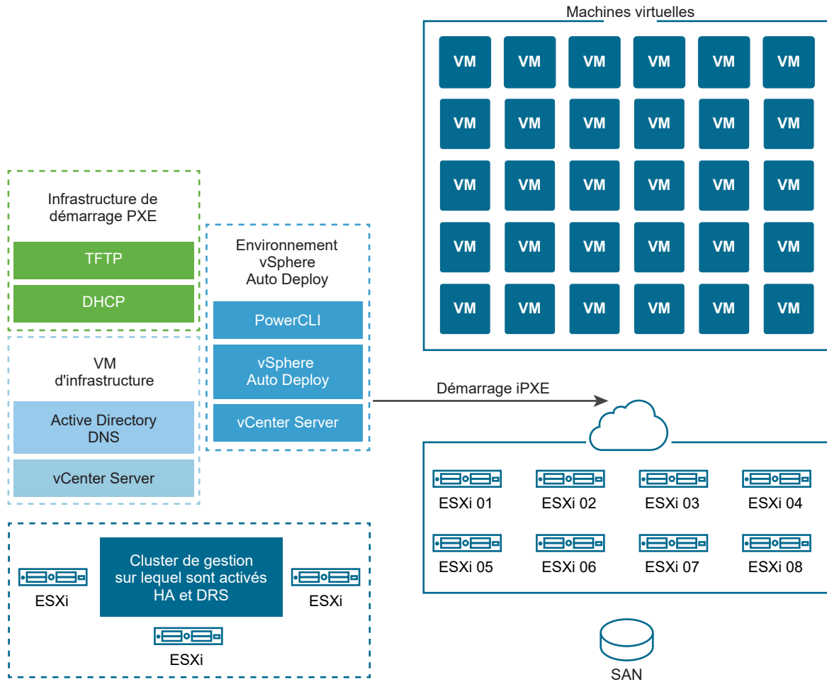
Figure 4-10. Infrastructure vSphere Auto Deploy à haute disponibilité
