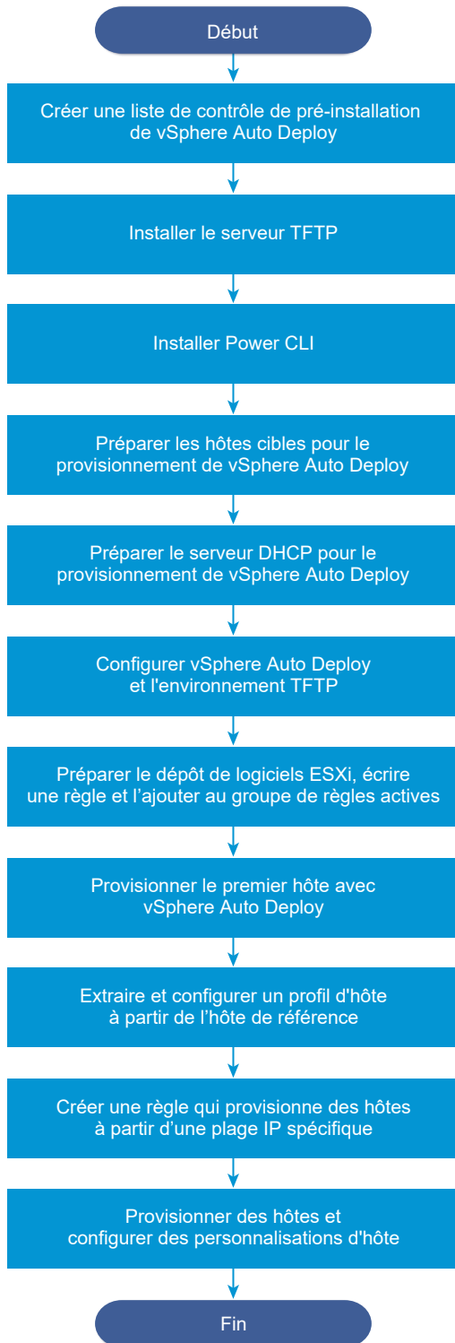
Figure 4-11. Workflow de configuration de vSphere Auto Deploy et de provisionnement d'hôtes
