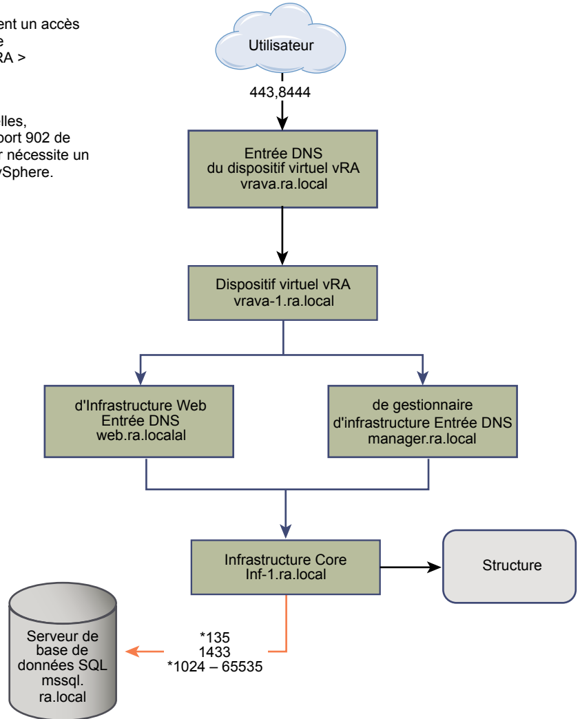
Figure 9-1. Encombrement minimal pour une petite configuration de vRealize Automation
