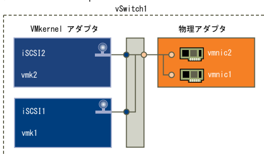
図 4-3. 1 つの vSphere 標準スイッチでの 1 対 1 のアダプタ マッピング
