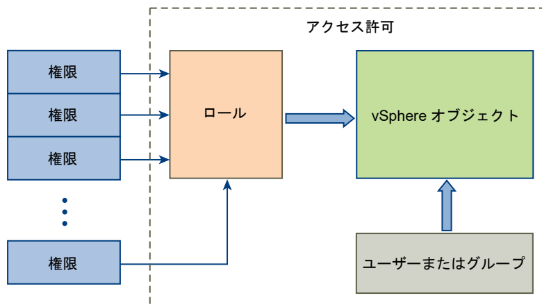
図 2-1. vSphere の権限
