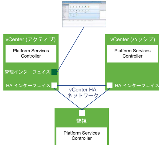
図 4-2. 組み込み Platform Services Controller を持つ vCenter HA
