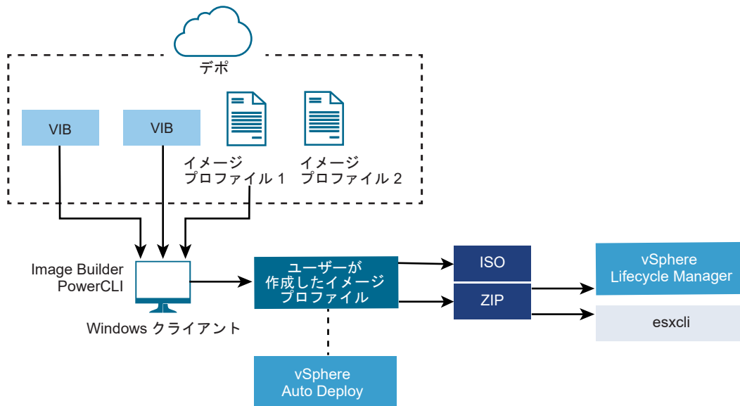
図 5-2. Image Builder のアーキテクチャ
