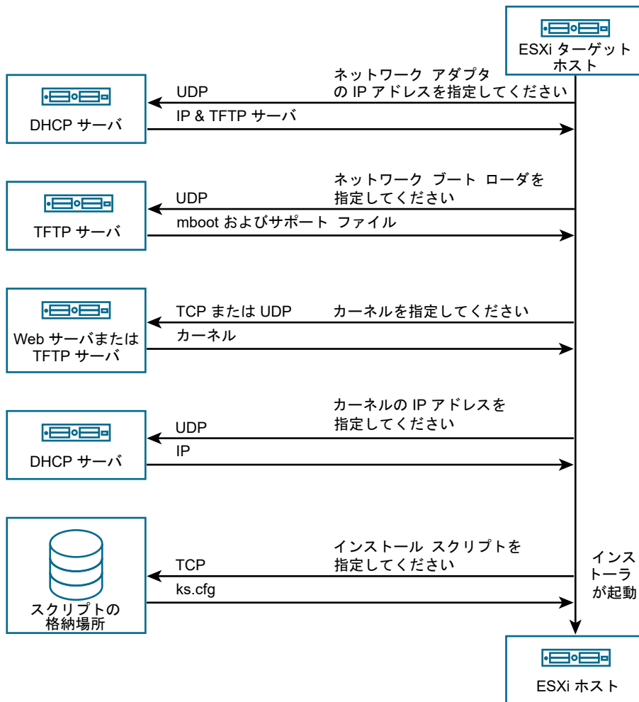
図 5-3. PXE ブートのインストール プロセスの概要
