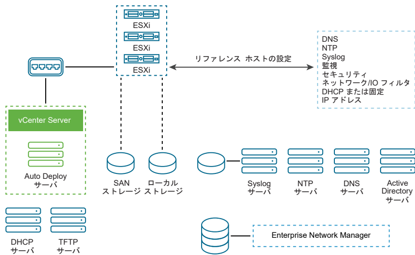
図 5-7. vSphere Auto Deploy のリファレンス ホストのセットアップ
