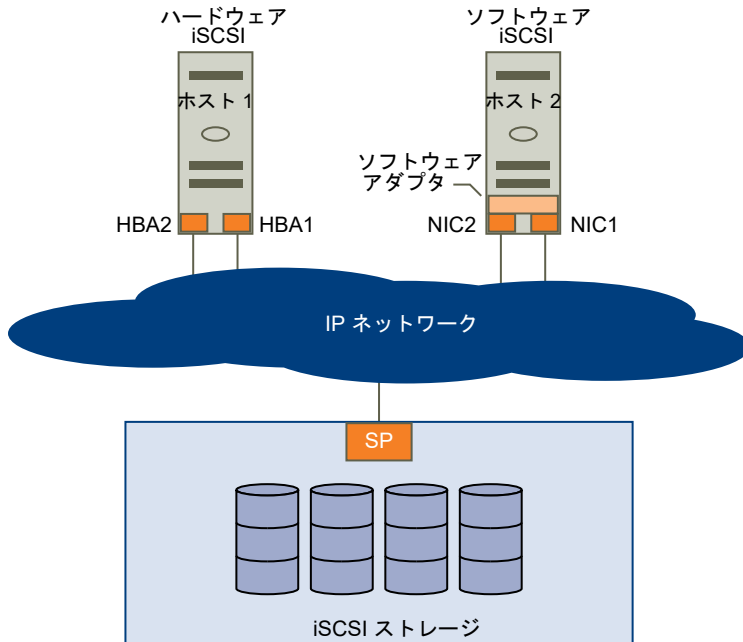
図 18-2. ホスト ベースのバス フェイルオーバー
