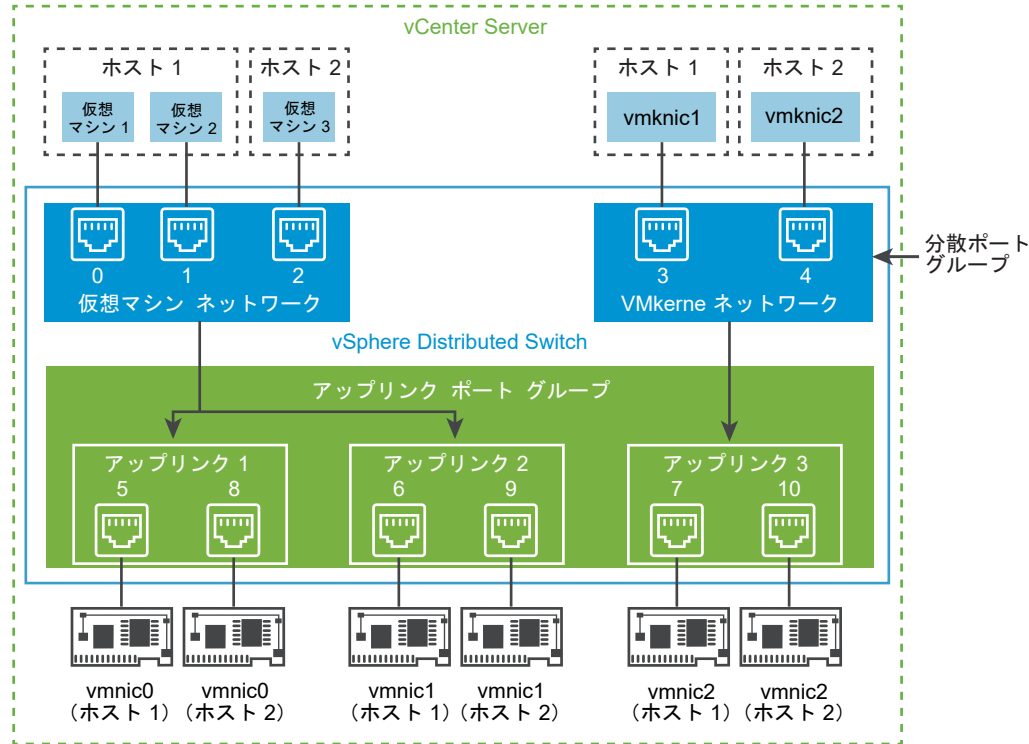
図 3-2. vSphere Distributed Switch の NIC チューニングおよびポートの割り当て
