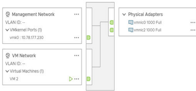
図 2-2. vSphere 標準スイッチのトポロジ ダイアグラム
