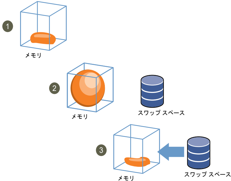
図 6-1. ゲスト OS のメモリ バルーン化
