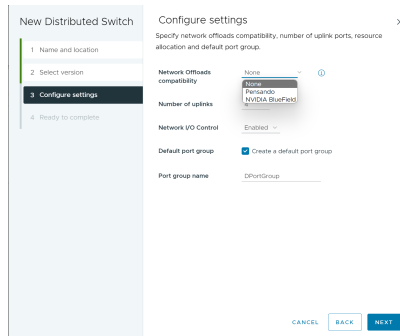
図 3-4. ネットワーク オフロードの互換性
