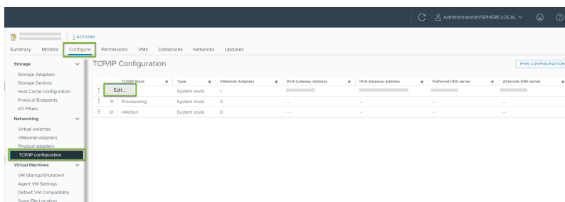
図 13-1. TCP/IP 設定
