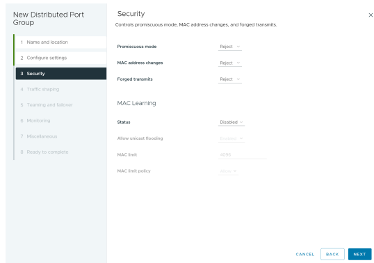
図 3-7. 新規分散ポートグループ - セキュリティ
