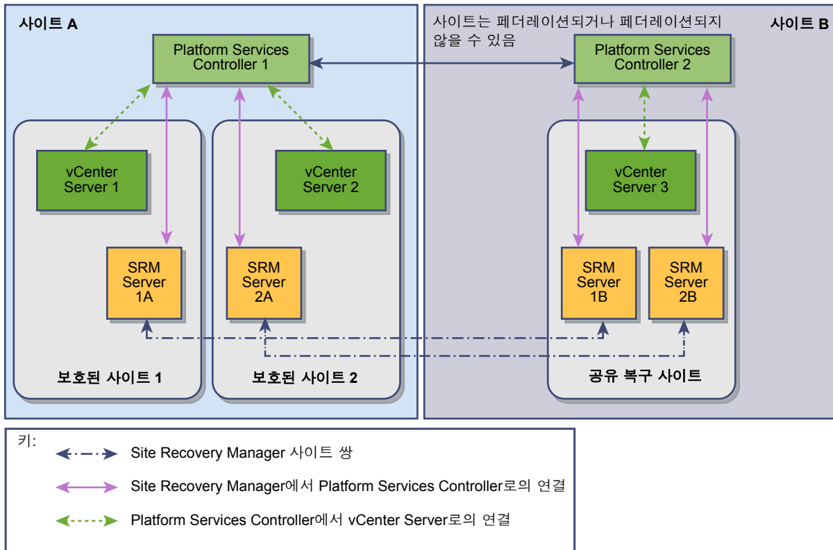
그림 9-2. 공유 복구 사이트 구성의 Site Recovery Manager
