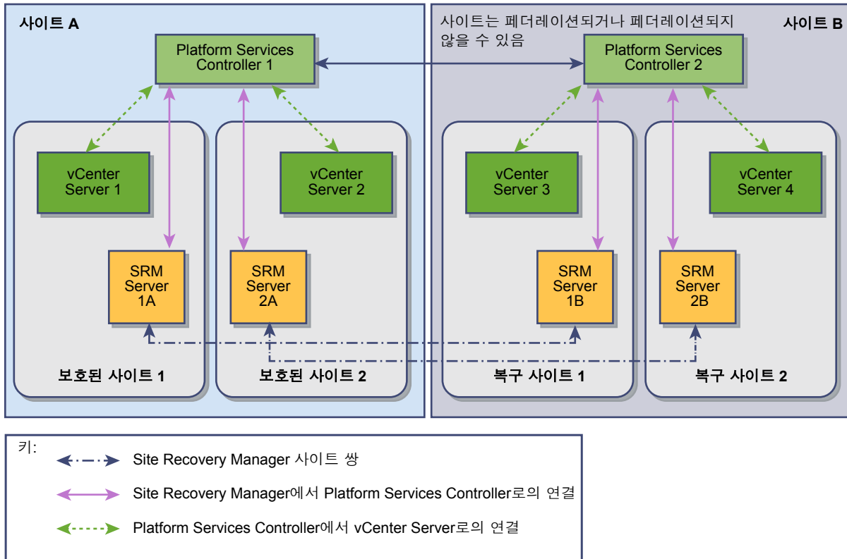
그림 6-2. Platform Services Controller 당 2개의 vCenter Server 인스턴스가 있는 2사이트 토폴로지의 Site Recovery Manager
