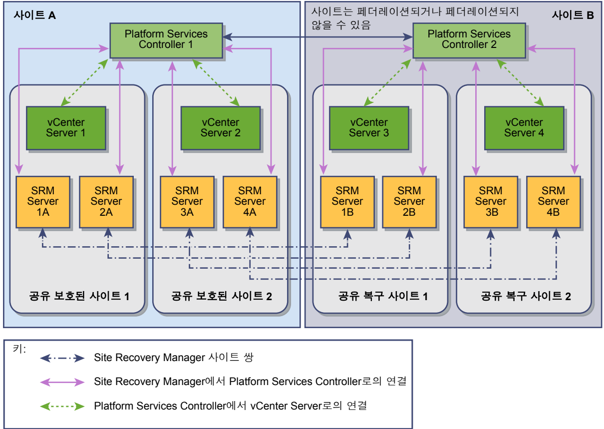
그림 10-3. 공유 보호된 사이트 및 공유 복구 사이트 구성의 Site Recovery Manager
