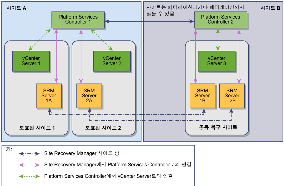
그림 10-2. 공유 복구 사이트 구성의 Site Recovery Manager
