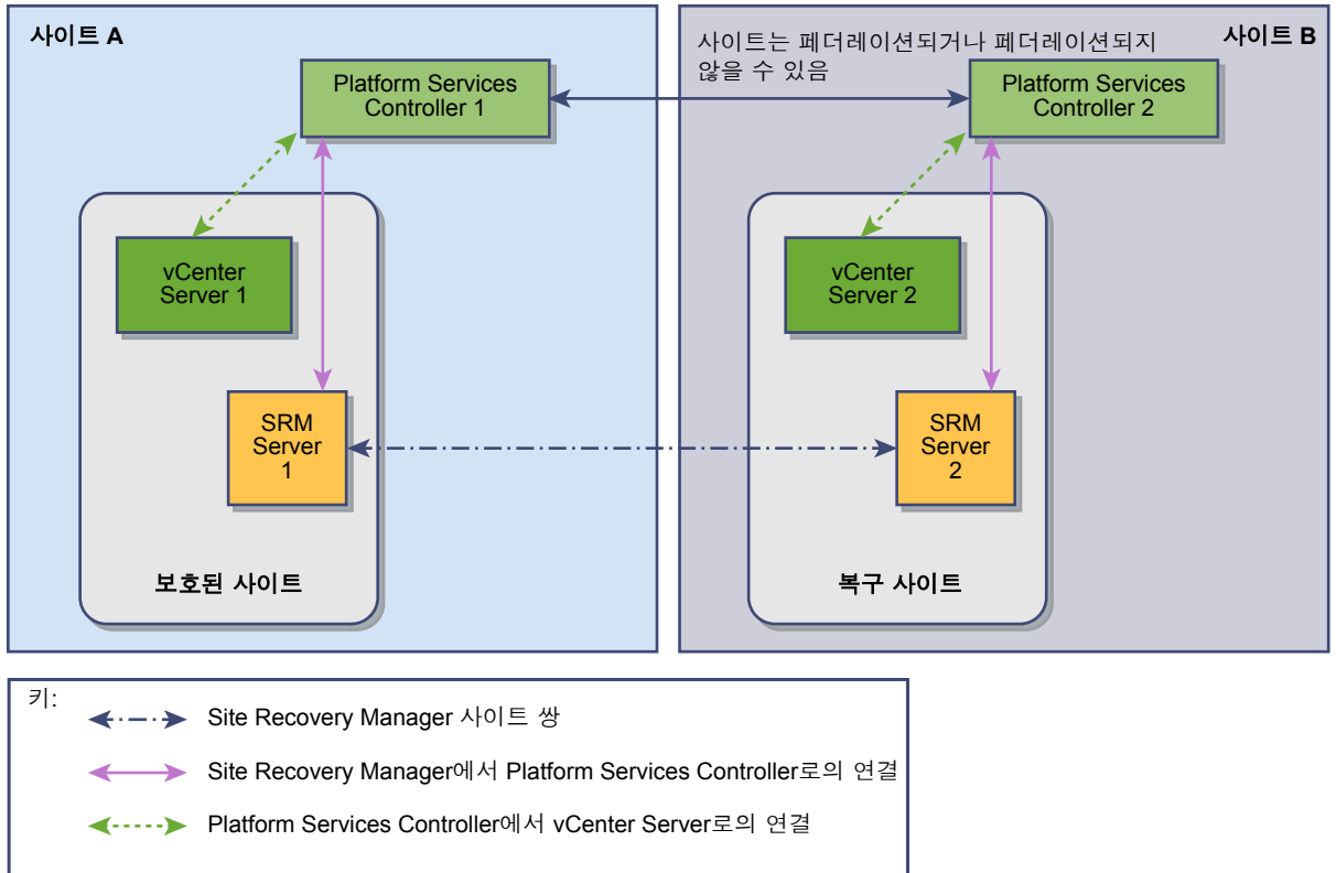
그림 6-1. Platform Services Controller 당 하나의 vCenter Server 인스턴스가 있는 2사이트 토폴로지의 Site Recovery Manager
