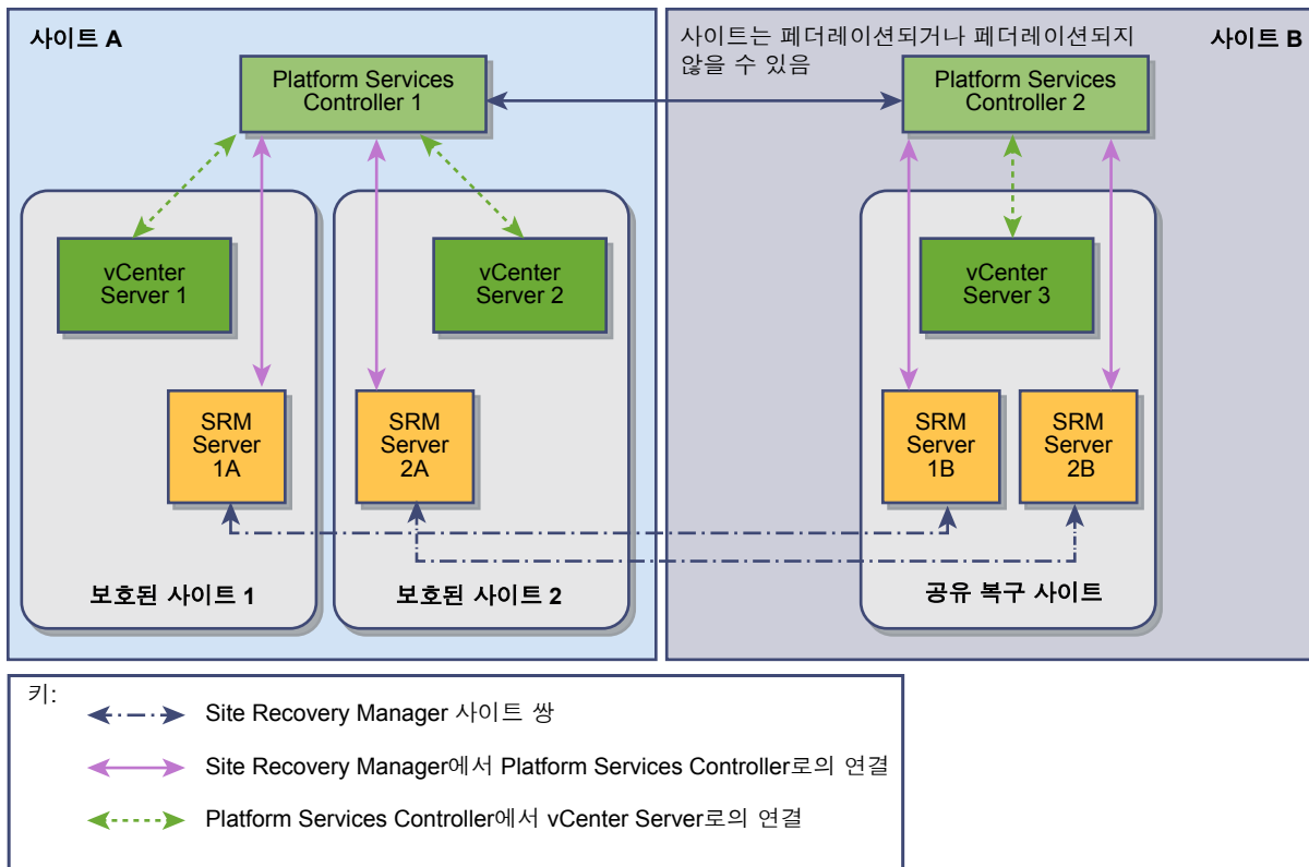
그림 10-2. 공유 복구 사이트 구성의 Site Recovery Manager
