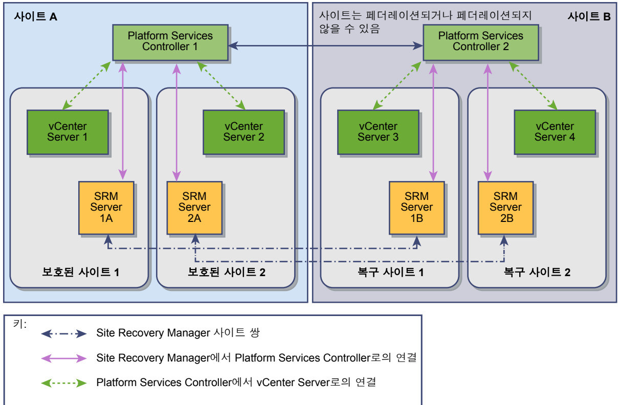
그림 6-2. Platform Services Controller 당 2개의 vCenter Server 인스턴스가 있는 2사이트 토폴로지의 Site Recovery Manager
