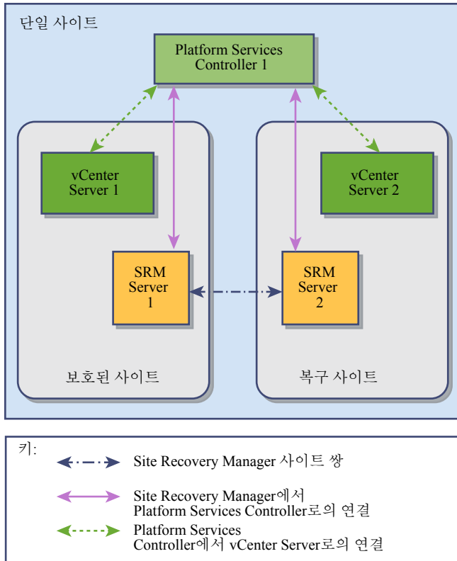
그림 6-3. 공유 Platform Services Controller 가 있는 단일 사이트 토폴로지의 Site Recovery Manager
