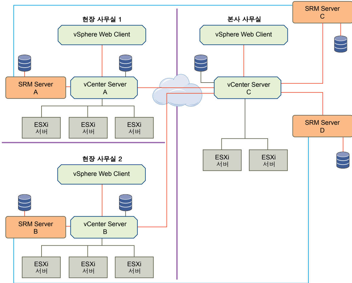
그림 10-1. 공유 복구 사이트 구성에서 Site Recovery Manager 사용 예 보호된 사이트 공유 복구 사이트
