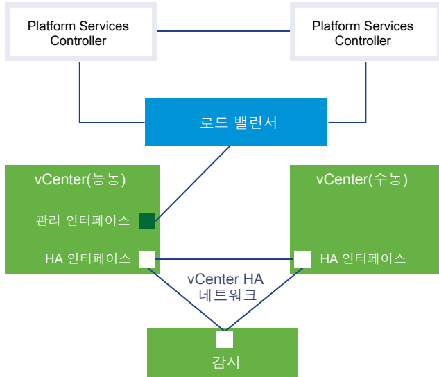
그림 4-3. 외부 Platform Services Controller 가 있는 vCenter HA
