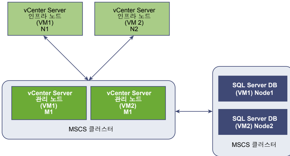
그림 5-1. vCenter Server 고가용성을 위한 MSCS 클러스터
