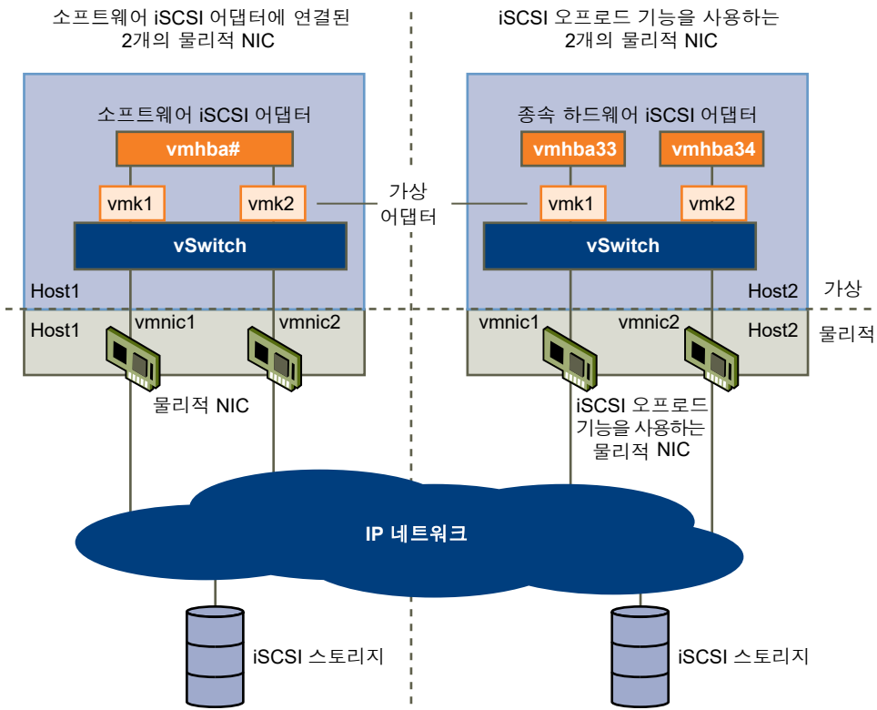
그림 11-1. iSCSI와의 네트워킹
