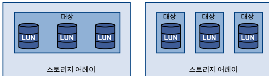
그림 10-1. LUN 표현과 비교되는 대상
