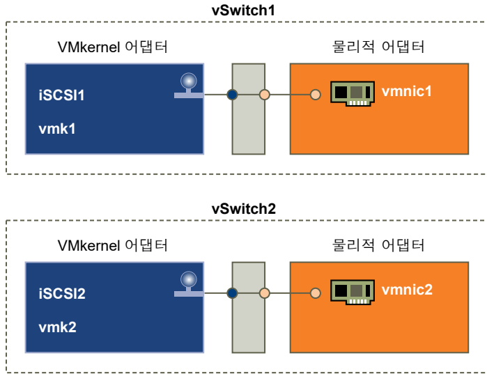
그림 11-2. 개별 vSphere Standard Switch에 대한 1:1 어댑터 매핑
