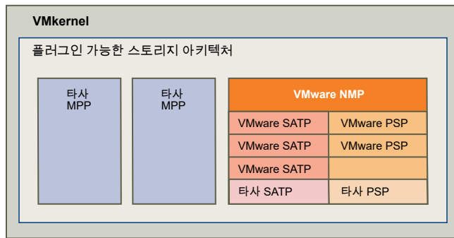
그림 18-5. 플러그인 가능한 스토리지 아키텍처
