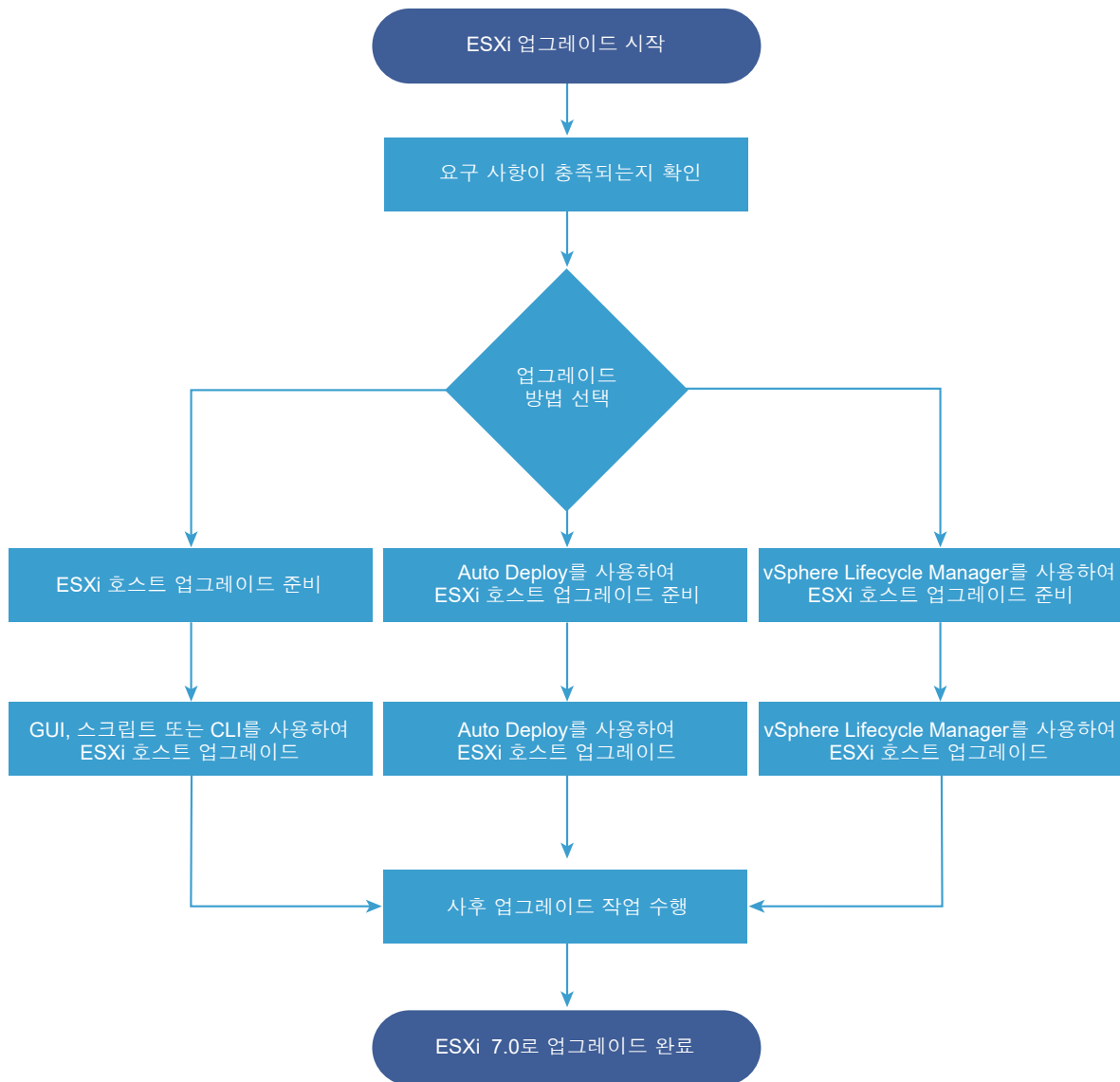
그림 2-2. ESXi 호스트 업그레이드 프로세스 개요
