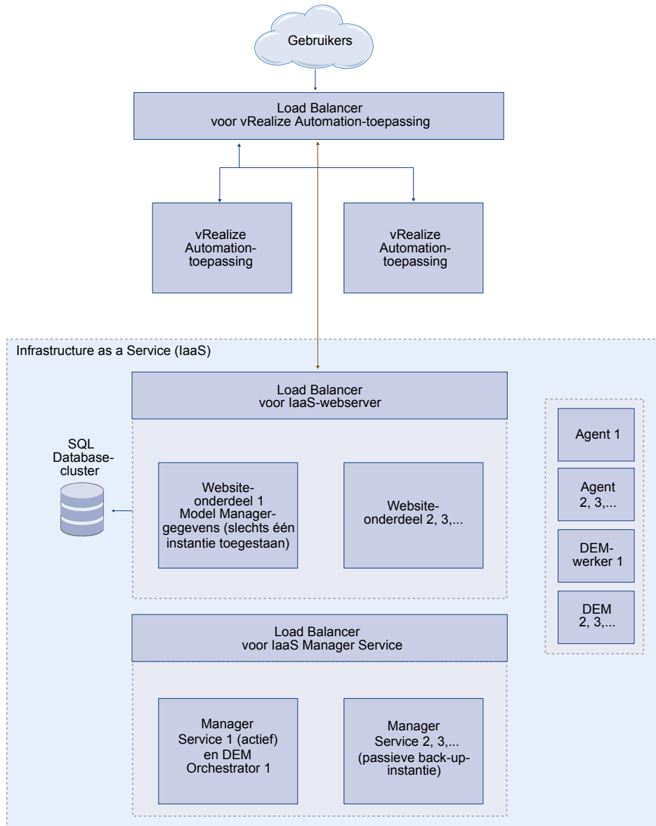
Figuur 1-1. Implementatieconfiguratie voor bedrijfsinstallaties
