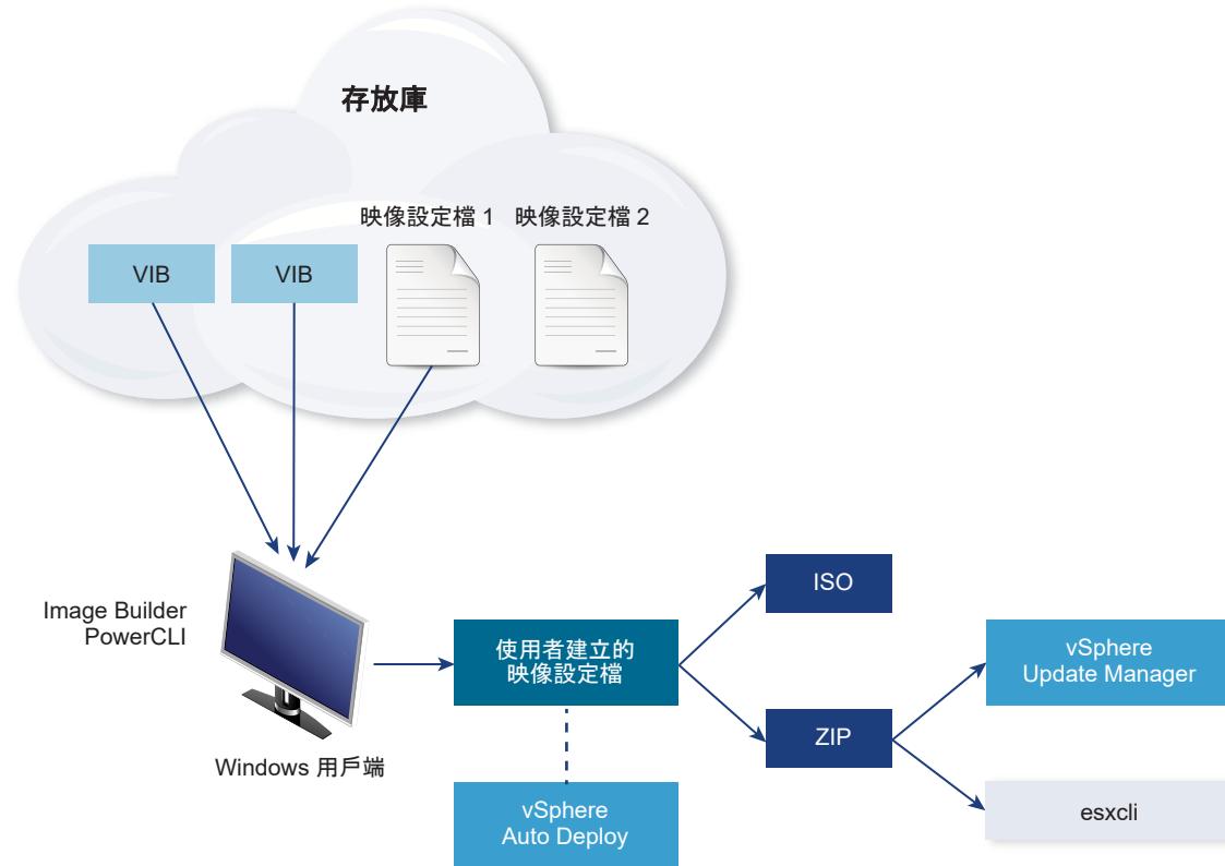
圖 5-2. Image Builder 架構
