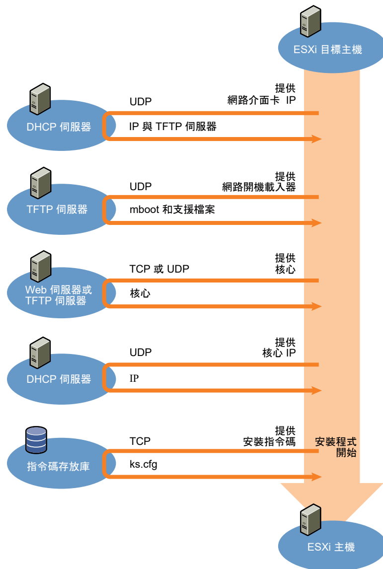
圖 5-3. PXE 開機安裝程序概觀
