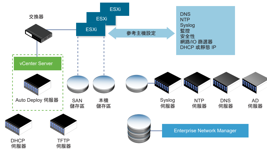
圖 5-7. vSphere Auto Deploy 參考主機設定
