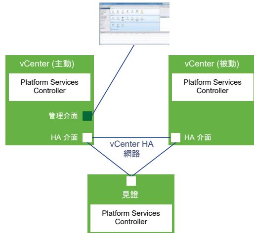
圖 4-2. 含內嵌式 Platform Services Controller 的 vCenter HA
