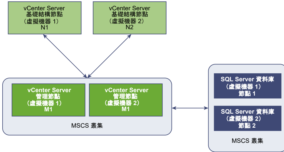
圖 5-1. 提供 vCenter Server 高可用性的 MSCS 叢集
