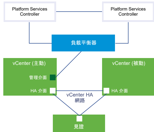
圖 4-3. 含外部 Platform Services Controller 的 vCenter HA
