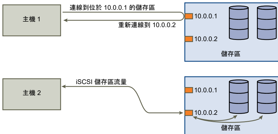
圖 18-3. 連接埠重新導向
