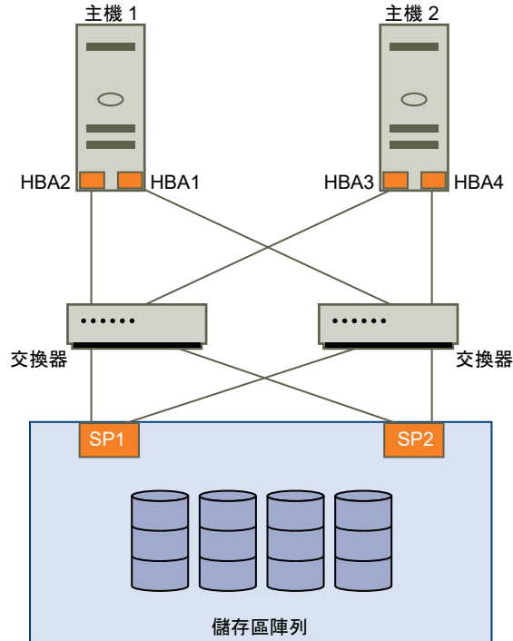
圖 18-1. 多重路徑和光纖通道容錯移轉
