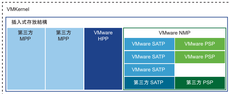
圖 18-5. 插入式存放結構
