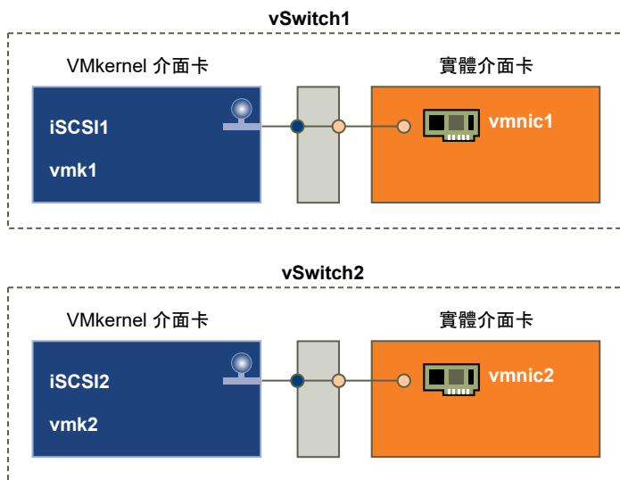
圖 11-1. 單獨 vSphere 標準交換器上的 1:1 介面卡對應
