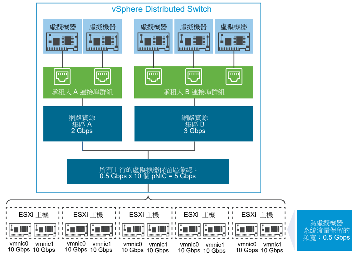
圖 11-1. vSphere Distributed Switch 上行之間的網路資源集區頻寬彙總
