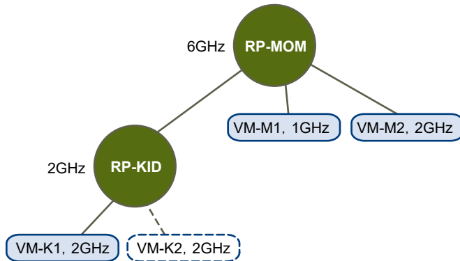
圖 10-4. 可擴充資源集區的許可控制：無法開啟電源
