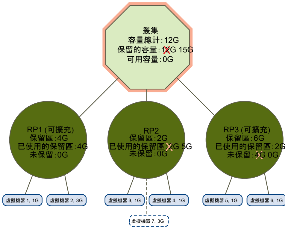
圖 13-4. 紅色叢集
