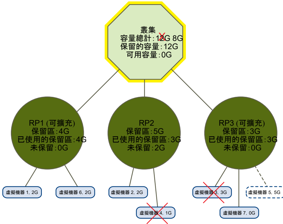
圖 13-3. 黃色叢集
