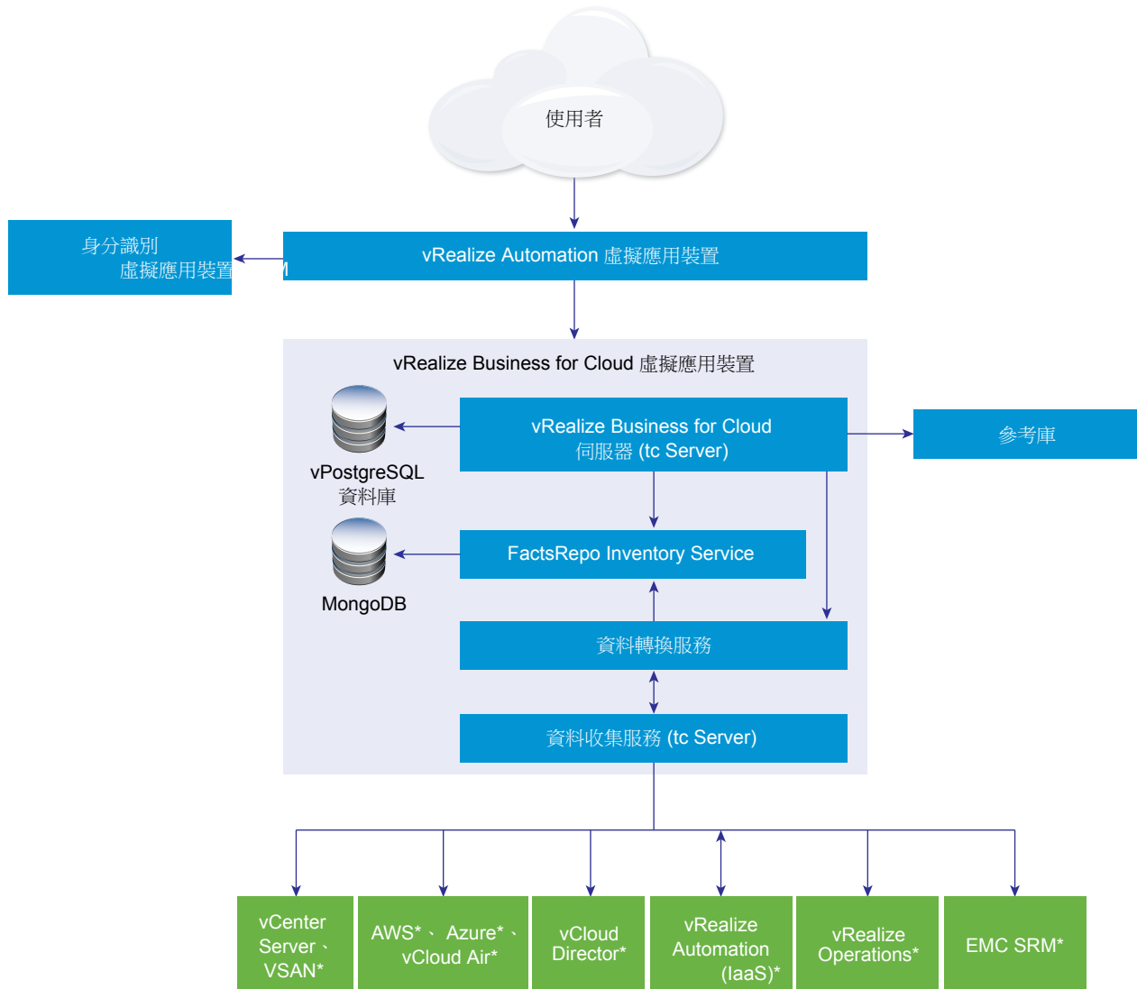
圖 1-1 vRealize Business for Cloud 架構
